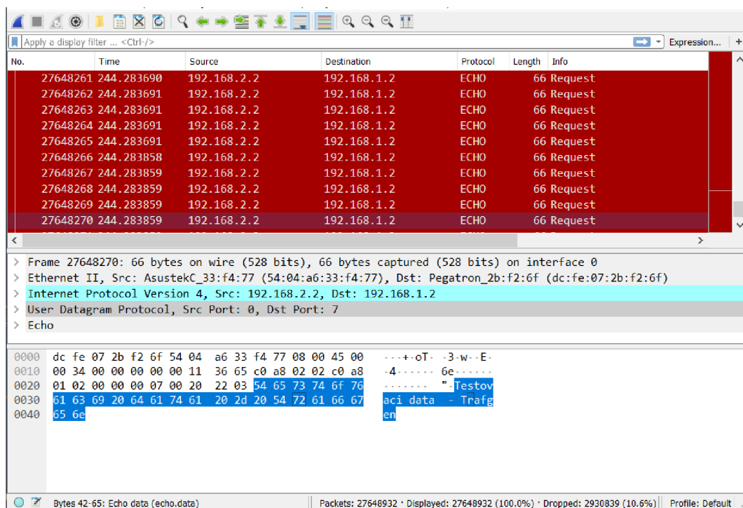
Obr. 4.10 Wireshark při druhém útoku
