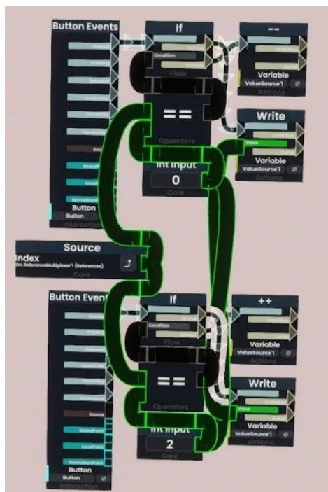
Obrázek 28: ProtoFlux funkce: Switching Logic Zdroj: autor
