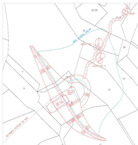
Obr. 31: Výkres z projektové dokumentace Poldru 2 zřízeného v rámci PPO v Přisece. Na obrázku se je možné vidět homogenní hráz, bezpečnostní přeliv, výpustný objekt, plocha stálého nadržení, meandrující potok a dvě tůně (Šindler 2015)
