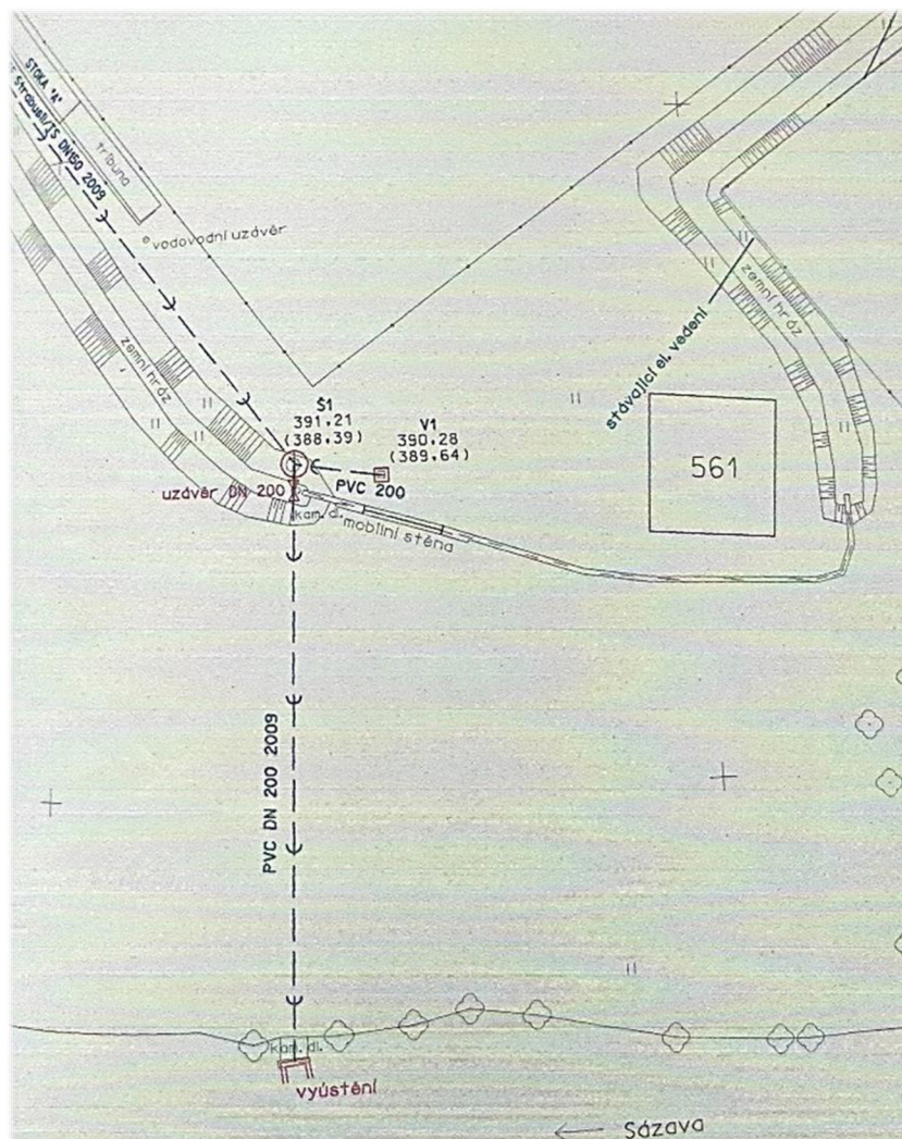
Obr. 34: Výkres PPO na fotbalovém hřišti ve Světlé nad Sázavou (Drupos – projekt 2018)
