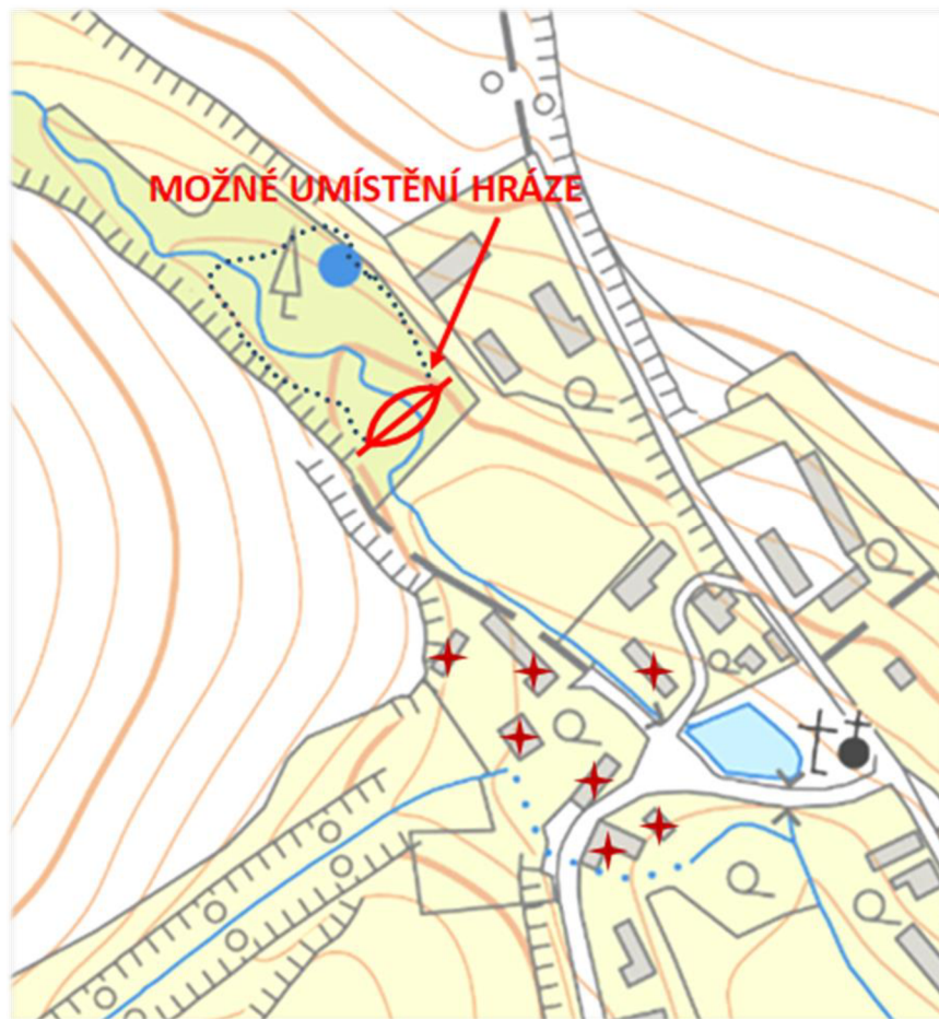
Obr. 45: Vyznačení možného umístění hráze poldru. V místě historicky zaniklého rybníka s protrženou hrází. Nachází se na bezejmenném vodním toku (tok č.1) v nezastavěné oblasti. Šest domů a přilehlých pozemků je sužováno povodněmi (vyznačeno znakem hvězdy) ( https://www.voda.gov.cz/ ; autor 2023).
