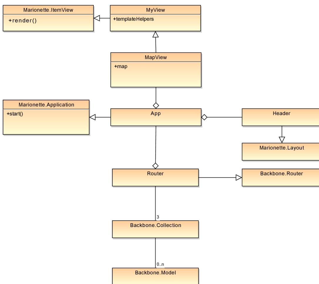
Obrázok C.1: Diagram tried aplikácie. Neobsahuje všetky triedy – chýbajú skoro všetky pohľady a zobrazená je iba jedna kolekcia.
