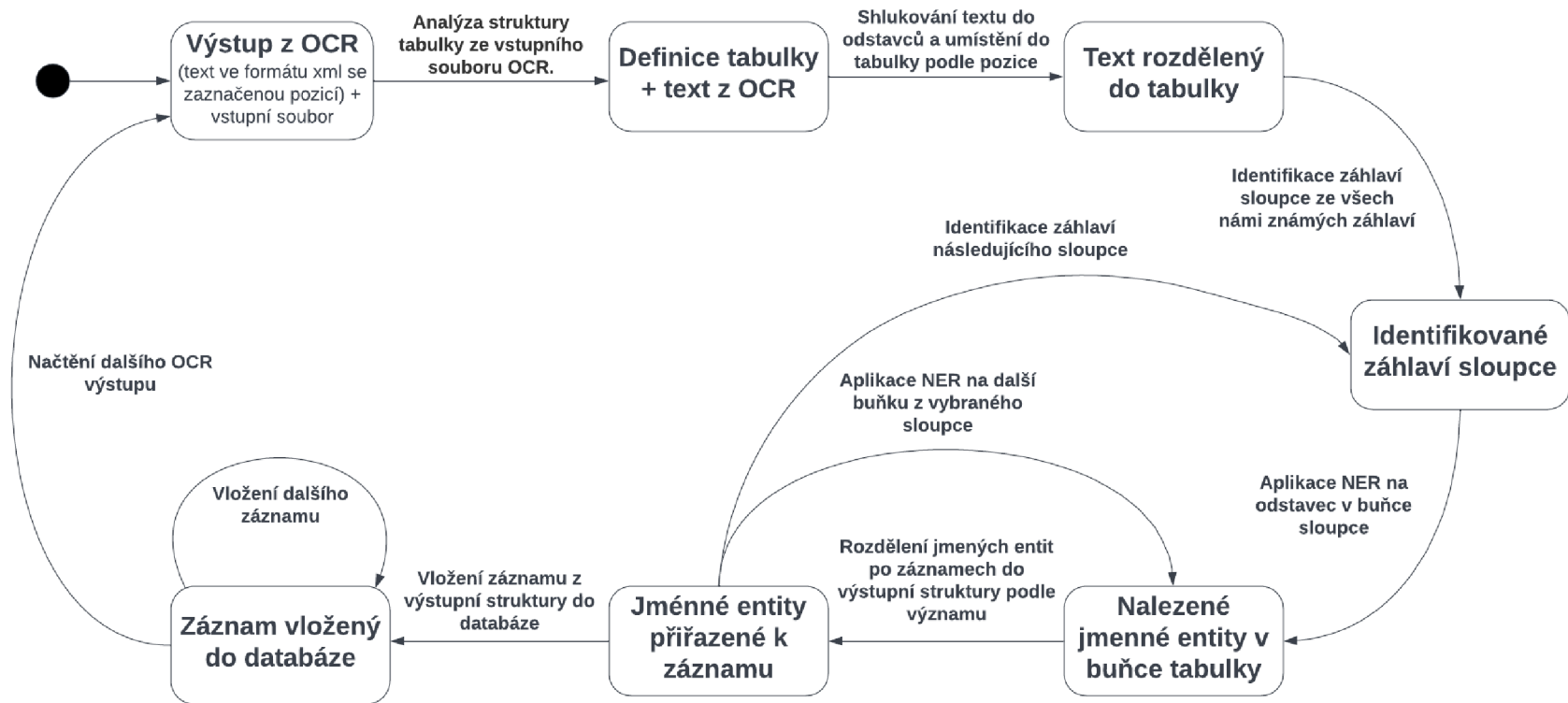
Obrázek 3.1: Stavový automat navržené aplikace
