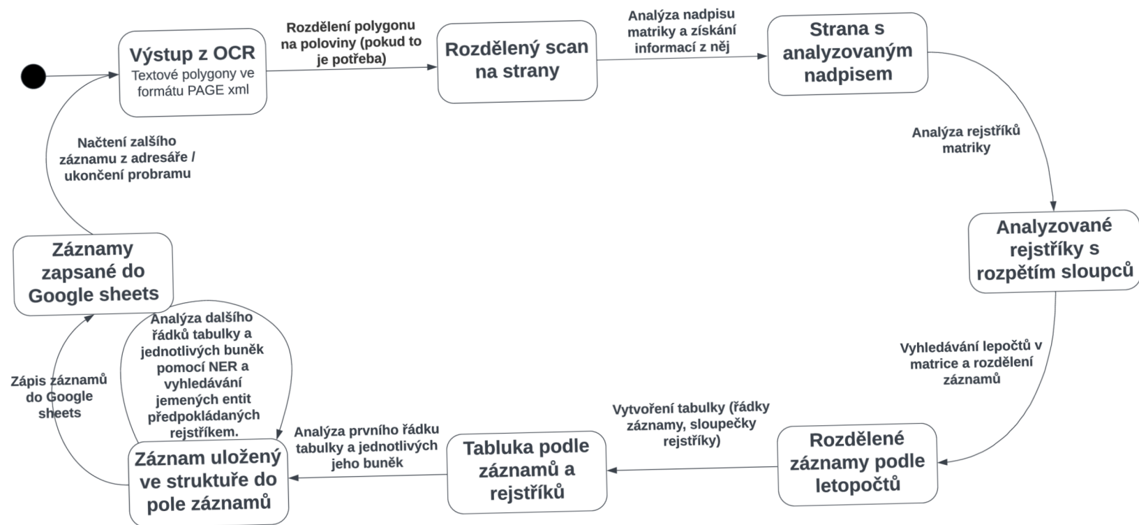
Obrázek 4.3: Stavový automat výsledné aplikace
