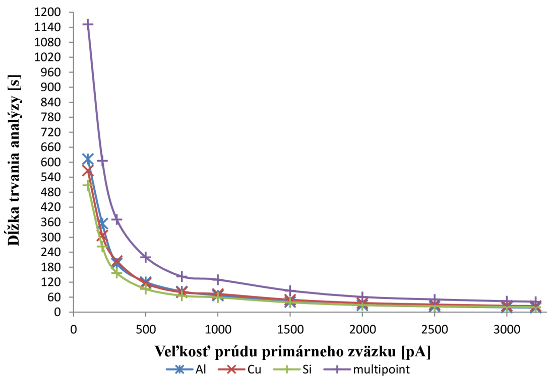
Obr. 5.18: Závislosť dĺžky trvania jednotlivých analýz na veľkosti prúdu primárneho zväzku
