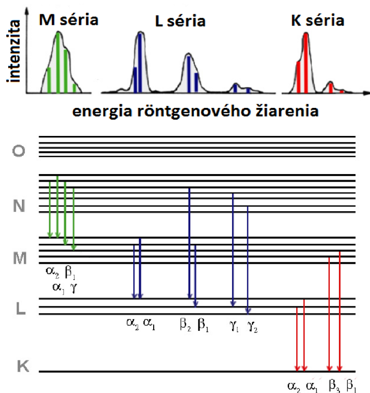
Obr. 4.4: Skupiny spektrálnych čiar a ich intenzity [1]
