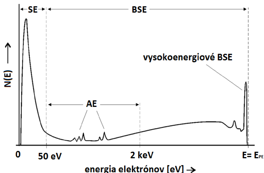
Obr. 3.3: Schematické energetické spektrum elektrónov emitovaných po dopade primárnych elektrónov na povrch vzorky. SE - sekundárne elektróny, BSE – spätne odrazené elektróny, AE – Augerové elektróny [9]
