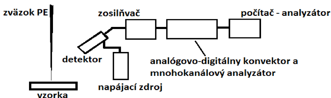
Obr. 4.1: Bloková schéma energiovo disperzného röntgenového spektroskopu [3], [6]
