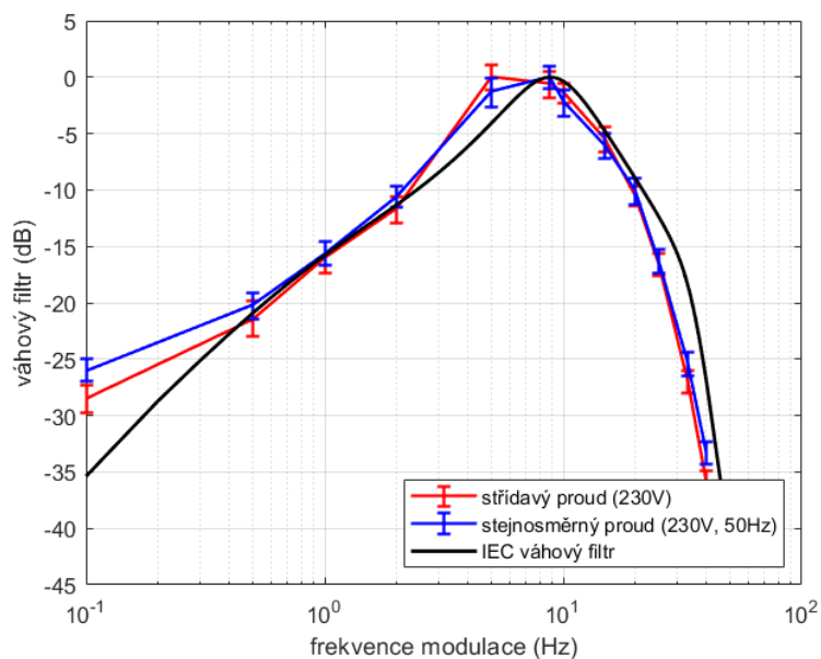
Graf 8.5: Porovnání naměřených dat s tvarem váhového filtru IEC napět'ového flickrmtru
