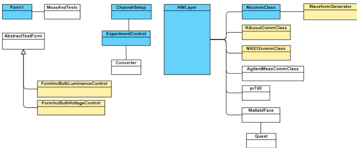
Obrázek 5: Zjednodušený diagram tříd, kde bílé označené třídy byly vytvořeny před touto prací, modré byly v rámci práce rozšířeny, žluté byly kompletně vytvořeny v rámci práce
