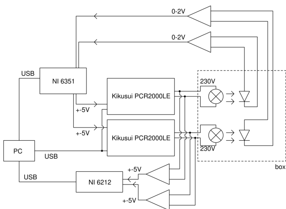
Obrázek 4: Zapojení hardwaru
