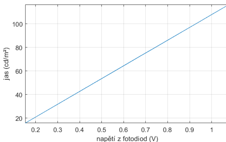
Graf 6.2: Závislost jasu na napětí z fotodiod
