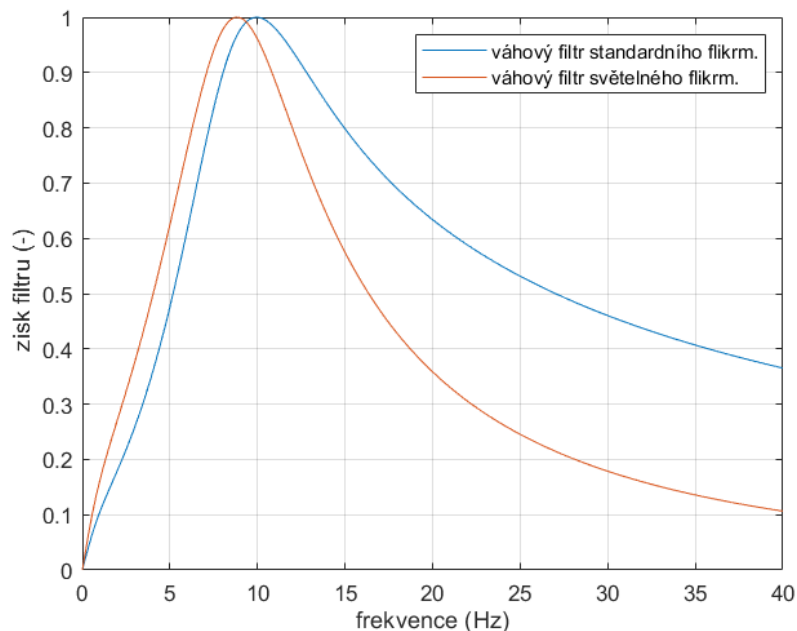
Graf 2.1: Porovnání normalizovaných váhových filtrů
