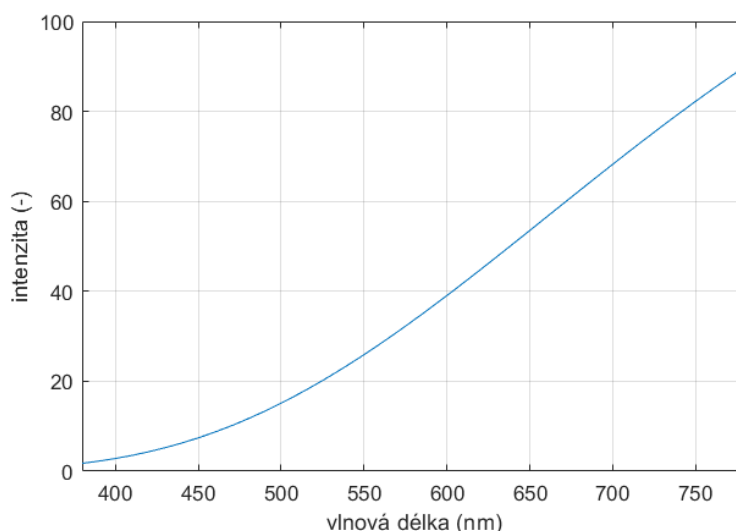
Graf 1.1: Ukázka spektra dle Planckova zákona
