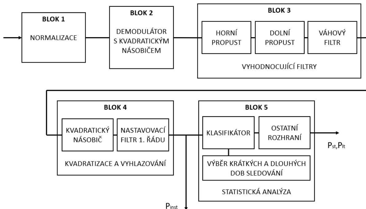
Obrázek 1: Schéma napěťového flikrmetru [2]
