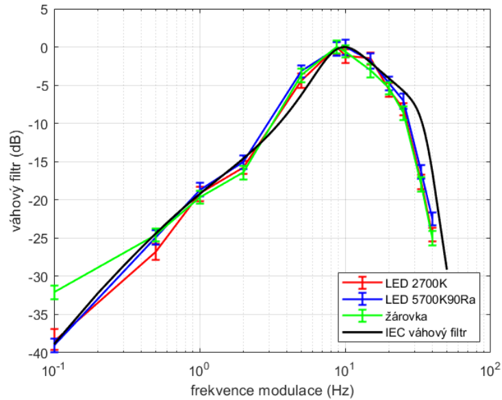
Graf 8.2: Porovnání naměřených dat s tvarem váhového filtru IEC světelného flikrmetru
