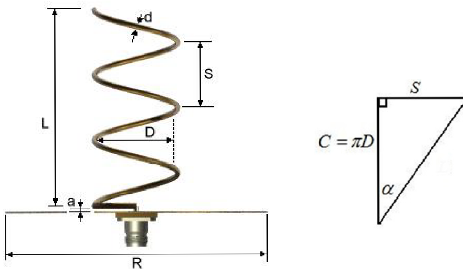
Obr. 39 Návrhové rozmery helix antény [4]
