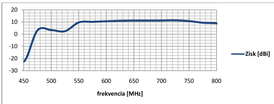
Obr. 44 Graf závislosti zisku helix antény na frekvencii - simulácia
