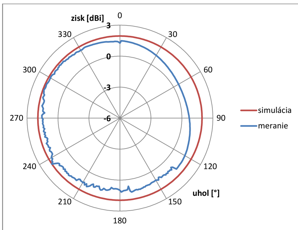
Obr. 31 Vyžarovacia charakteristika koaxiálnej antény v horizontálnej rovine
