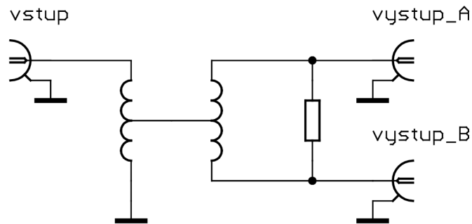
Obr. 13 Pridanie impedančného transformátora do obvodu rozbočovača
