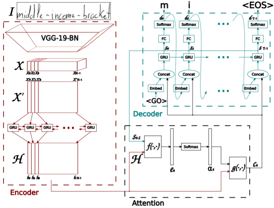
Obr. 2.5: Architektúra modelu, ktorý predstavil Kang a spol., zobrazuje hlavné použité komponenty a ich vzájomné prepojenie. Prevzaté z [22].
