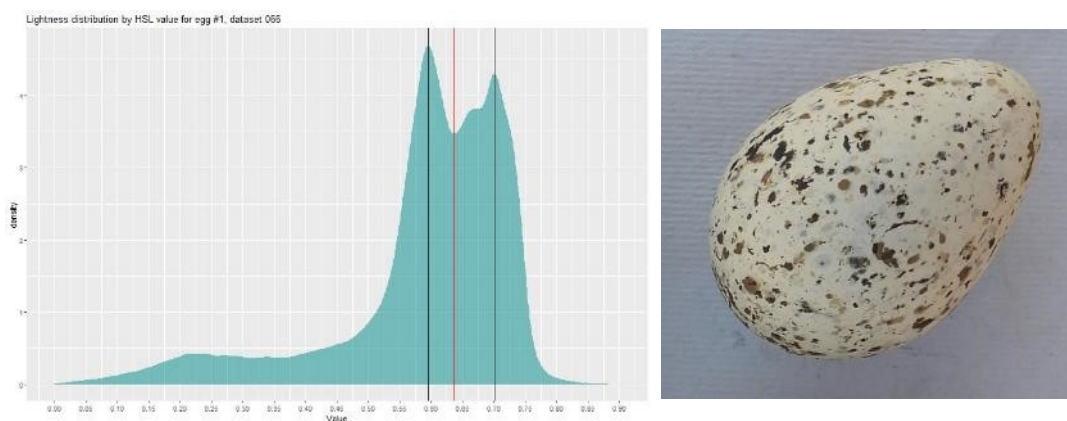
Obrázek 3 - Ukázka špatně určeného lokálního minima. Zde došlo k chybnému určení rozdělojících vrcholů z důvodu malého množství tmavých pixelů, kvůli výskytu pouze drobných skvrn na skořápce.
