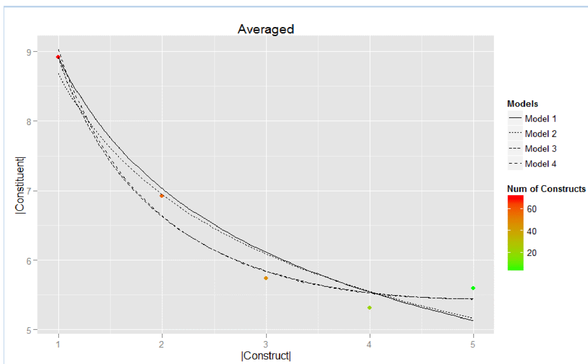
Obrázek 1 Grafické znázornění Menzerath-Altmannova zákona
