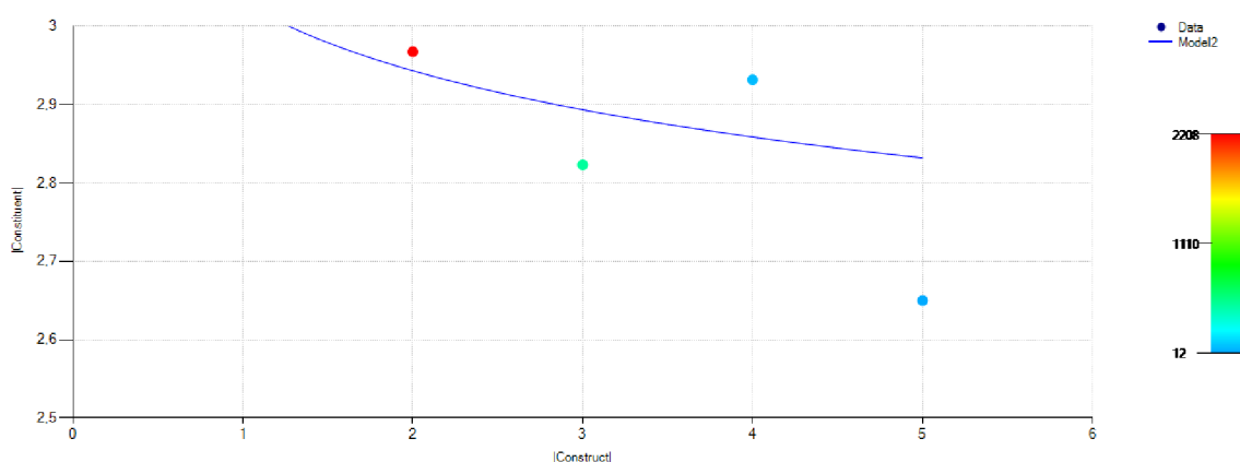
Obrázek 21 Experiment 1A: Grafická vizualizace pozorování uvedených v Tabulce 20 s proloženou regresní křivkou, Výběrový soubor 2: Yu Hua – Vítězství ženy pro jazykovou úroveň U3 (slovo měřené ve slabikách – slabika měřená v průměrném počtu grafémů) pro námi navržený způsob segmentace a po odebrání osobních zájmen on/ona/ono 他/她/它 tā
