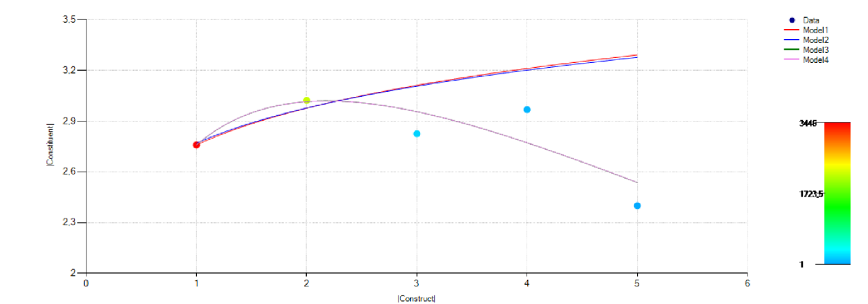
Obrázek 2 – Přílohy Grafická vizualizace pozorování uvedených v Tabulce 12 s proloženou regresní křivkou, Výběrový soubor 2: Yu Hua – Vítězství ženy pro jazykovou úroveň U3 (slovo měřené ve slabikách – slabika měřená v průměrném počtu grafémů)
