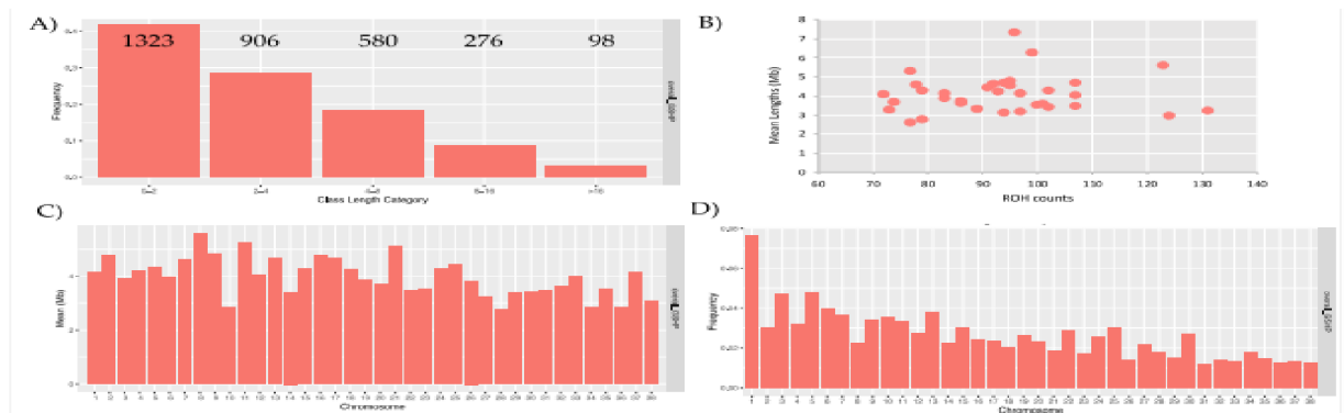
Graf 3 - graf štatistík o dĺžkach nástupu homozygotnosti (ROH). A) Frekvencie a počty ROH pre každú triedu dĺžky; B) Vzťah medzi počtom a priemernou celkovou dĺžkou (Mb) ROH u každého psa; C) stredná dĺžka (Mb) pre každý chromozóm; D) Frekvencie ROH na chromozómoch
