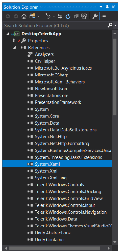
Obrázek 6 - Reference projektu
