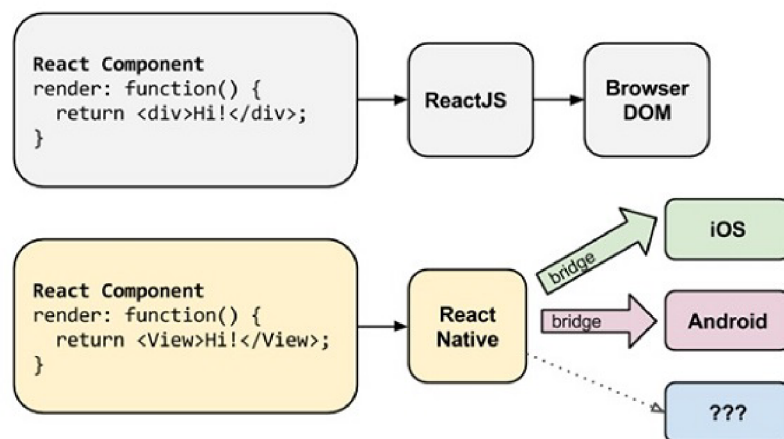
Obrázek 3.6: Způsob vykreslování v React Native. Převzato z: [9]
