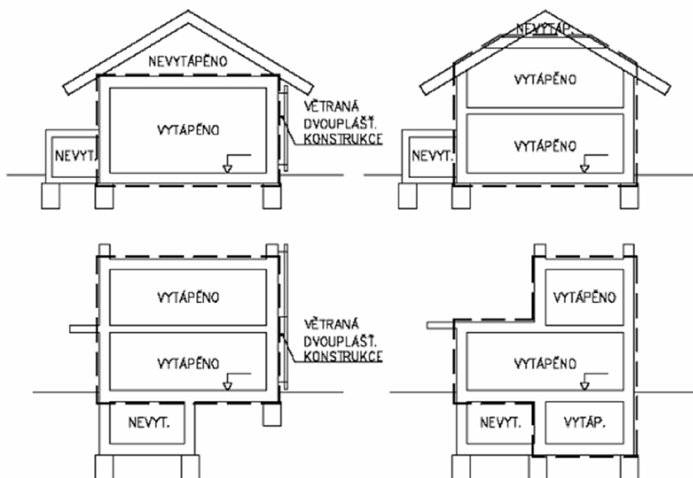
Obrázek 5 - Objemový faktor budovy [47]
