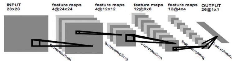
Obrázek 2.10: Příklad sítě užívající skryté konvoluční a pooling vrstvy. Vstupní obrázek o velikosti 28 \times 28 pixelů prochází přes tři konvoluční a dvě pooling vrstvy pro dosažení výsledného jednorozměrného vektoru. Převzato z [15].
