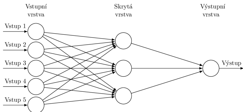
Obrázek 2.6: Obecný model neuronové sítě
