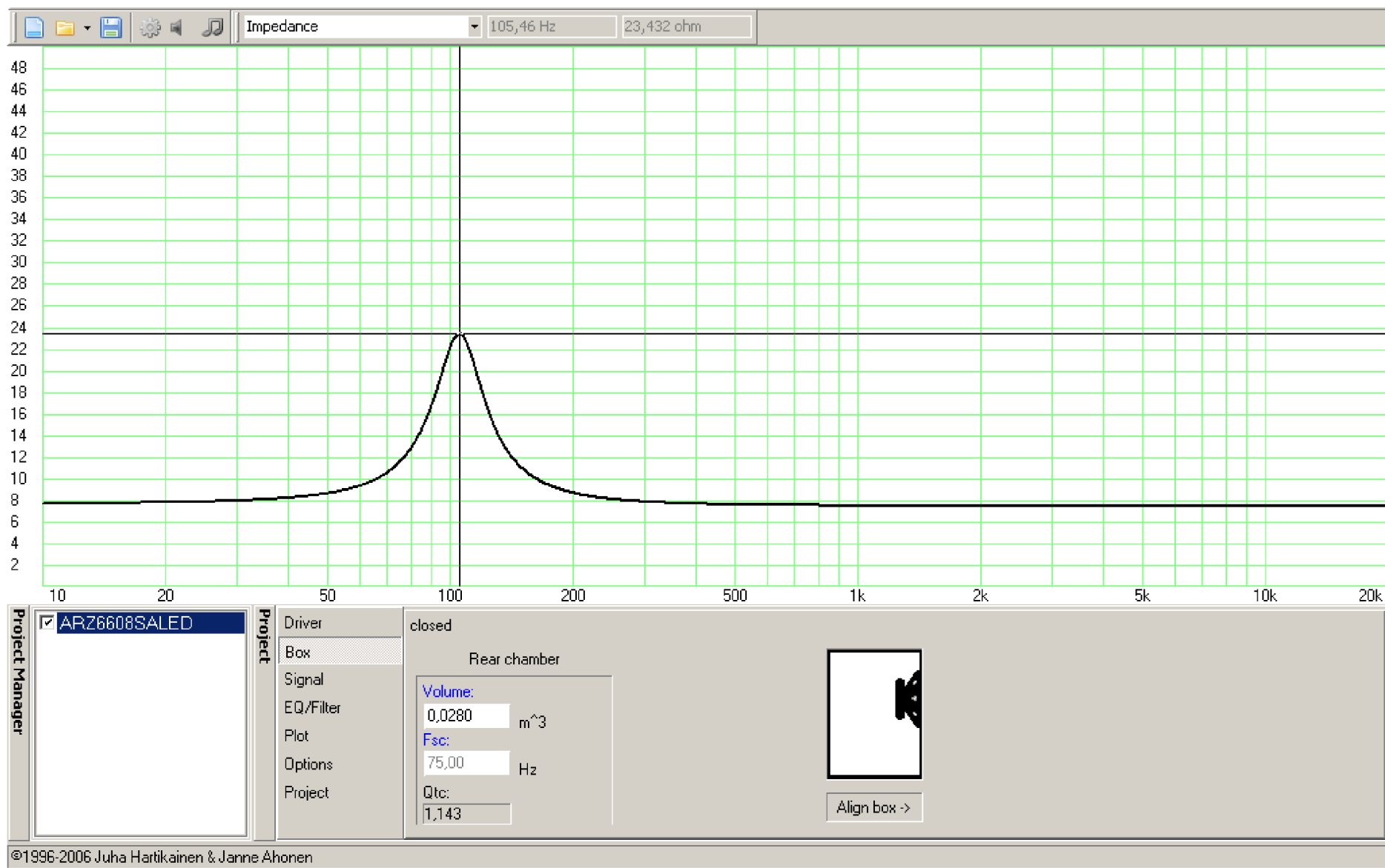
Příloha 4: Modulová impedanční charakteristika uzavřené ozvučnice, simulace WinISD 0.6
