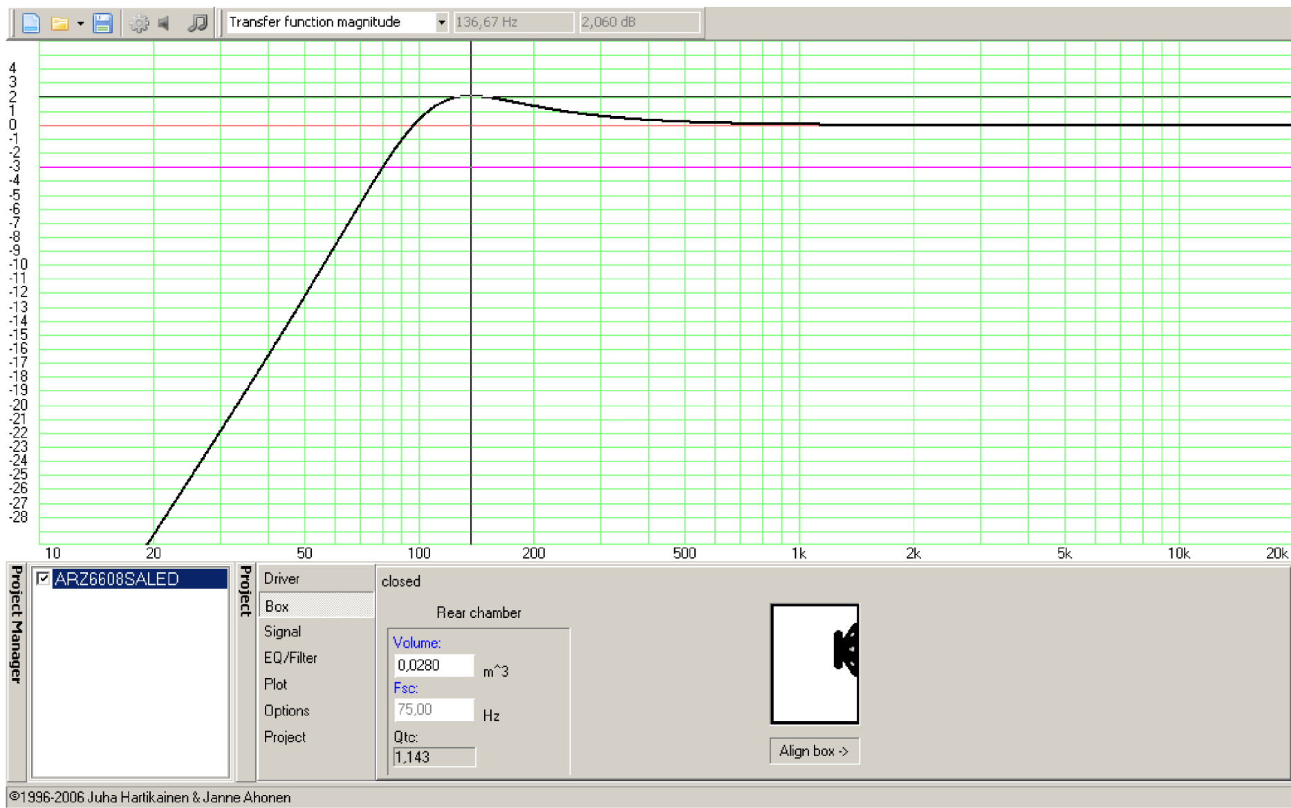
Příloha 3: Amplitudová kmitočtová charakteristika uzavřené ozvučnice, simulace ve WinISD 0.6
