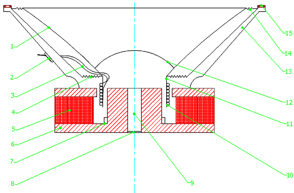
Obr. 1.1: Konstrukce elektromagnetického reproduktoru (klasická koncepce).
