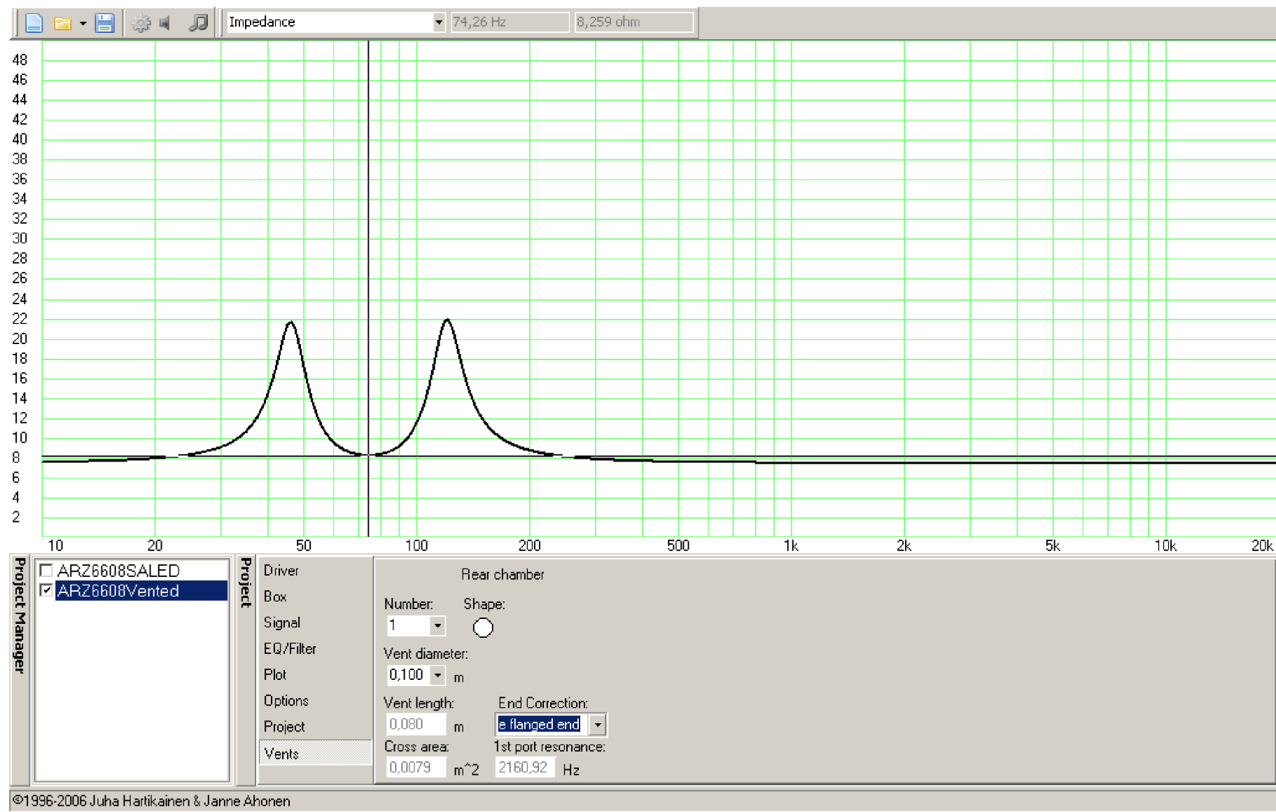
Příloha 6: Modulová impedanční charakteristika bassreflexové ozvučnice, simulace WinISD 0.6
