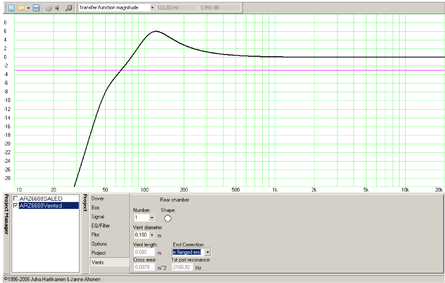
Příloha 5: Kmitočtová amplitudová charakteristika bassreflexové ozvučnice, simulace WinISD
