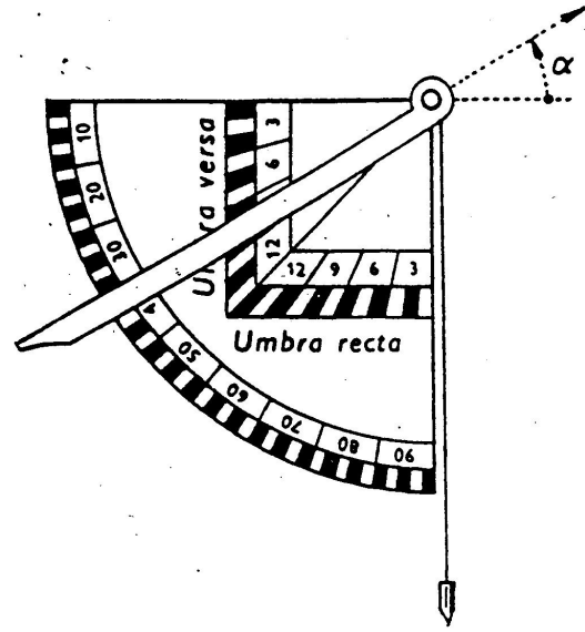
Obr. 1.3: Kvadrant
