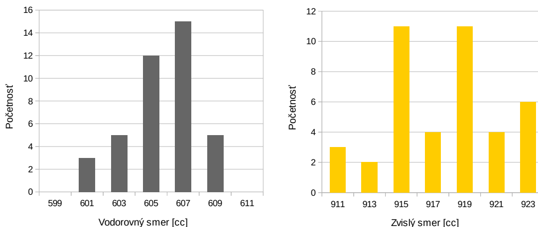
Obr. 3.4: Histogramy rozptylu pri manuálnom cielení (Topcon)
