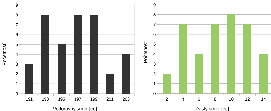
Obr. 3.6: Histogramy rozptylu pri manuálnom cielení (Leica)
