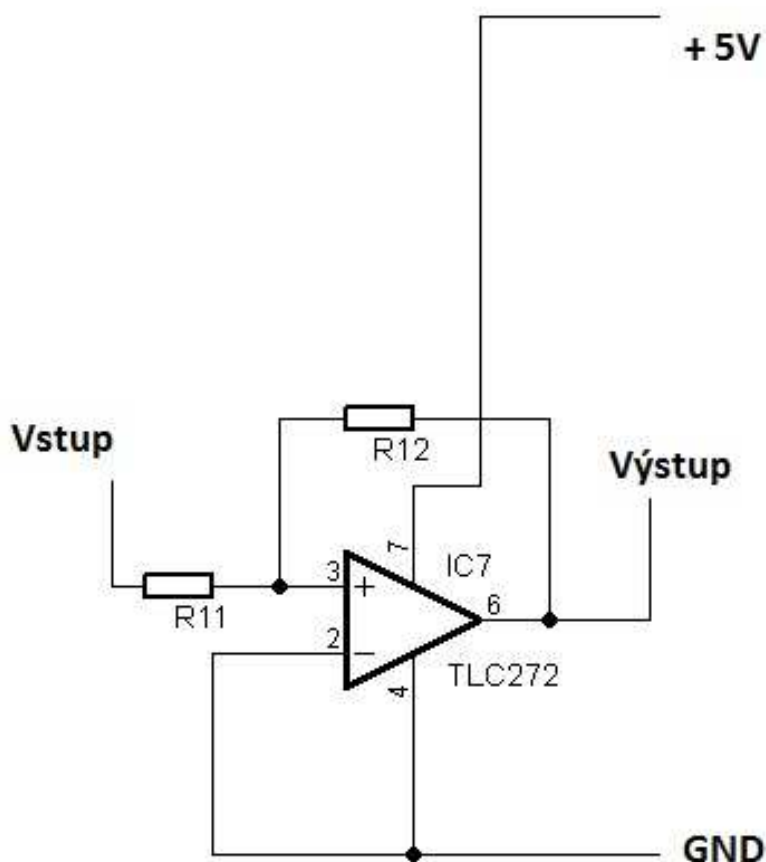
Obrázek č. 4.4 Schéma zapojení komparátoru s hysterezí v obvodu
