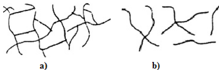
Obr. 2.6 Polymerní řetězce, a) termoset, b) termoplast, [12]
