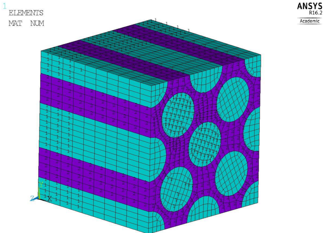
Obr. 4.3 Výpočtový model po přidání materiálu a vytvoření mesh sítě
