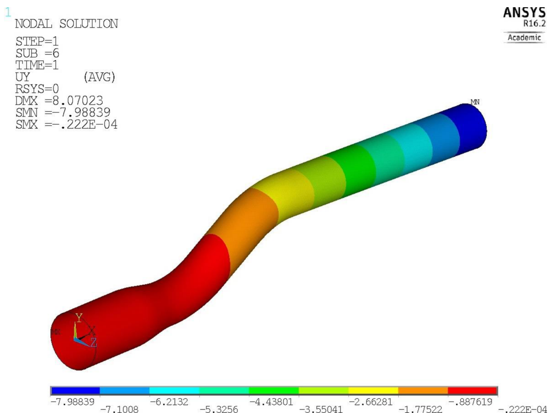
Obr. 6.6 Deformace modelu řídicítek ve směru osy Y
