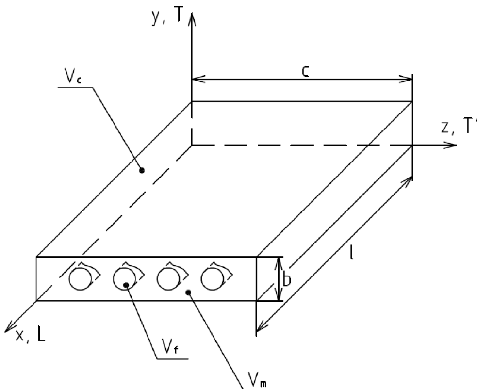
Obr. 4.1 Výpočtový model dlouhovláknového jednosměrného kompozitu, V_f – celkový objem vláken ve vzorku, V_m – celkový objem matrice ve vzorku, V_c – celkový objem vzorku, l – délka vzorku, b – tloušťka vzorku, c – šířka vzorku, překresleno z [1]
