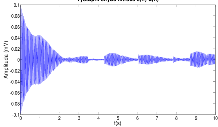
Obrázek 37. Chyba filtrace při frekvenci rušení 50,2 Hz Výstupní chyba filtrace e(n)-d(n)
