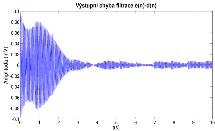
Obrázek 38. Chyba filtrace při frekvenci rušení 50,5 Hz Výstupní chyba filtrace e(n)-d(n)
