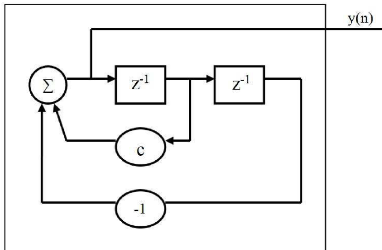
Obrázek 29. Rekurzivní rezonátor
