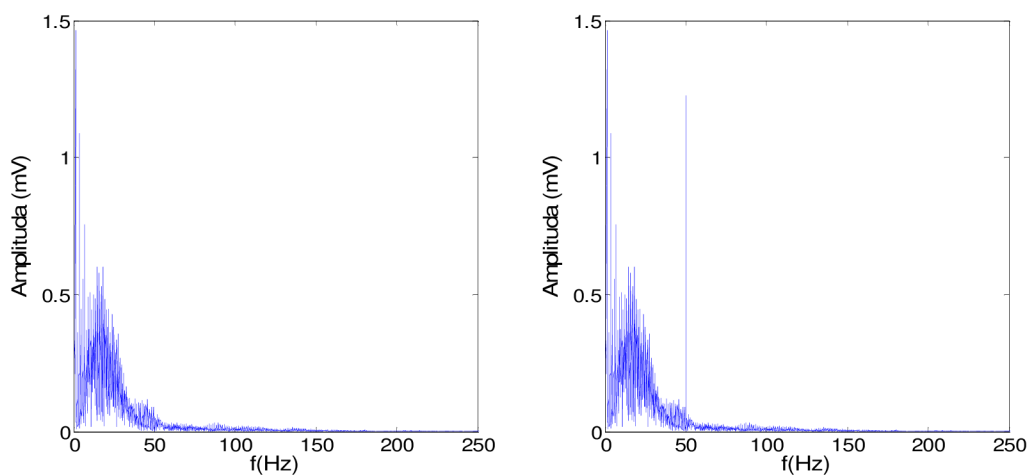
Obrázek 12. Amplitudové spektrum čistého a zarušeného signálu EKG
