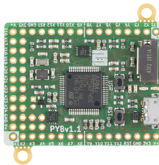
Obrázek 3.7: Modul Pyboard
