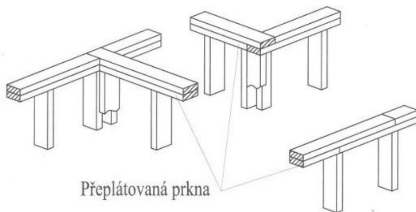
OBRÁZEK Č. 4: PROPOJENÍ RÁMU TBF KONSTRUKCE (KUKLÍK, 2005) ZLEVA: PŘÍČKOVÉ, ROHOVÉ, BĚŽNÉ
