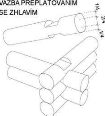
OBRÁZEK Č. 3: VARIANTY VAZEB (VENKOVSKÝ DŮM, 2022)
