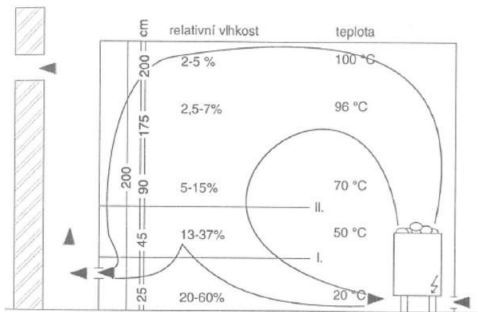
OBRÁZEK Č. 13: PŘENOS TEPLA VZDUCHEM (KRIŠ, 1998)
