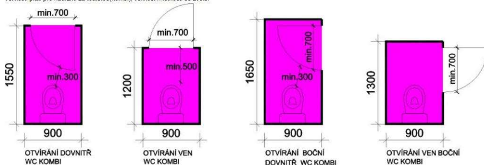
OBRÁZEK Č. 11: MINIMÁLNÍ SVĚTLÉ ROZMĚRY ZÁCHODOVÉ KABINY (ROBUST, 2023)
