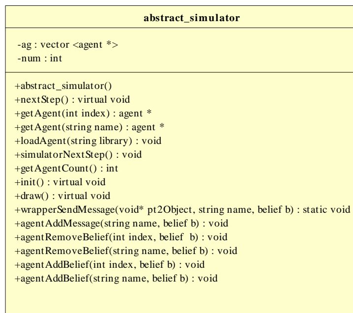
Obr. 4.6: Implementace simulátoru.
