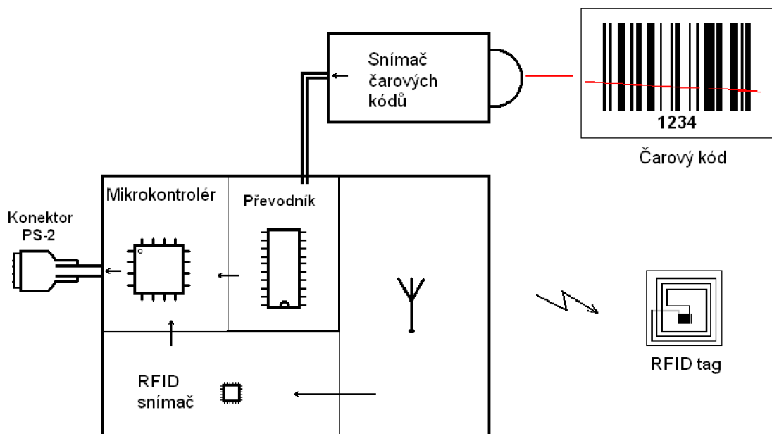
Obr. 5.1 Názorné zapojení bloků čtečky kódů.
