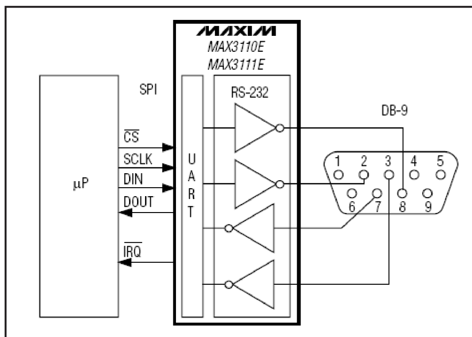
Obr. 5.7 Typické zapojení obvodu MAX3110.
