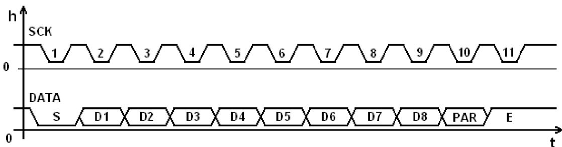
Obr. 5.4 Časový průběh PS-2 komunikace slave > master.
