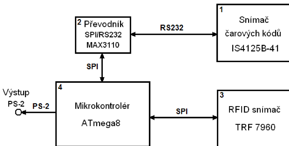
Obr. 5.2 Blokové schéma zařízení.
