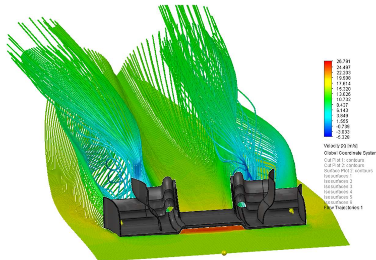
Obr. 43 3D vizualizácia prúdenia rýchlosti vzduchu - pohľad zhora [42]
