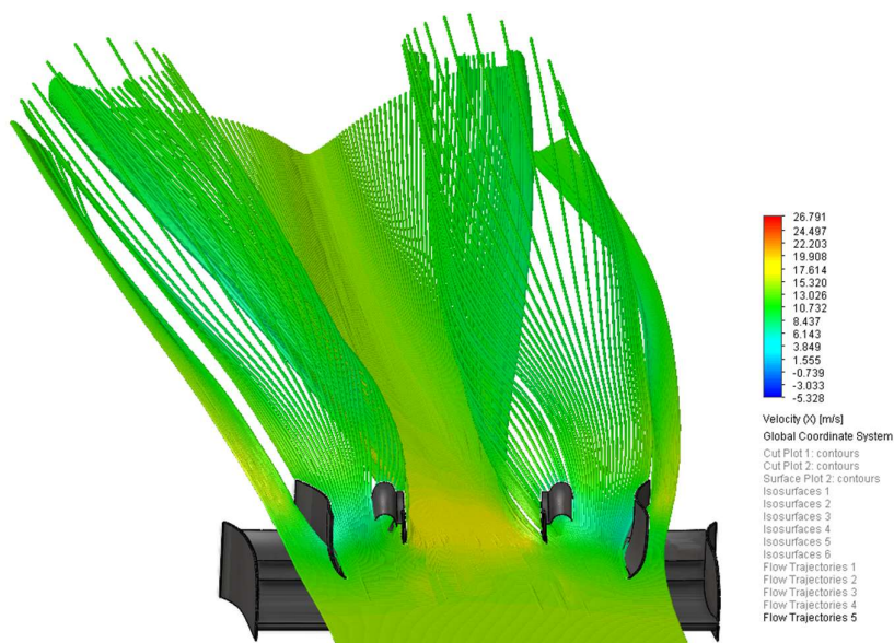
Obr. 45 Vizualizácia prúdenia cez vertikálne klapky - pohľad zhora [42]
