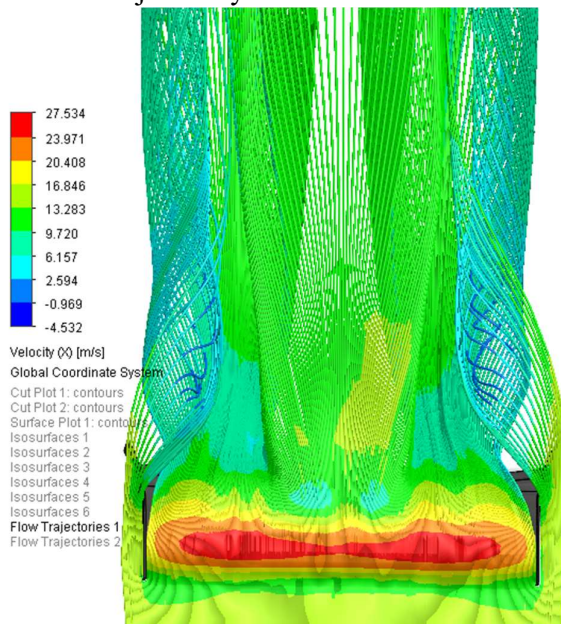
Obr. 52 Vizualizácia prúdenia spodnej strany krídla varianta 2 pohľad zdola [42]
