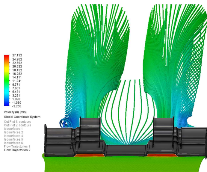
Obr. 59 3D vizualizácia prúdenia rýchlosti vzduchu varianta 3 [42]
