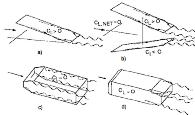
Obr. 6 Zobrazenie rôznych povrchov a následne vytváranie turbulentného prúdenia za nimi [9]
