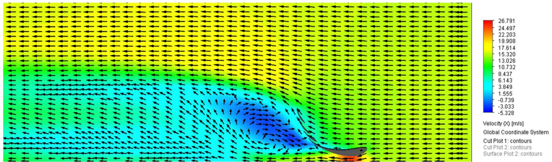
Obr. 42 Simulácia rýchlosti vzduchu v priereze s 3 lopatkami variantu 1 [42]
