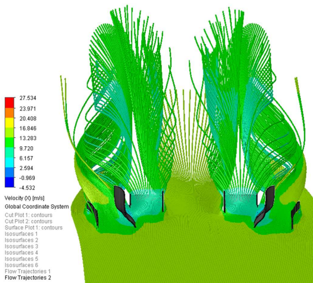
Obr. 53 Vizualizácia prúdenia cez vertikálne klapky varianta 2 pohľad zhora [42]
