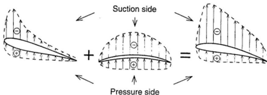
Obr. 11 Vytvárania tlaku na rôznych profiloch [13]
