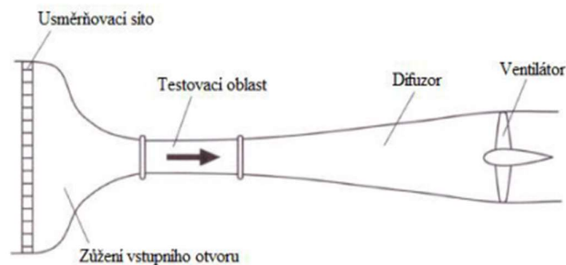
Obr. 28 Aerodynamický tunel s otvoreným systémom [38]
