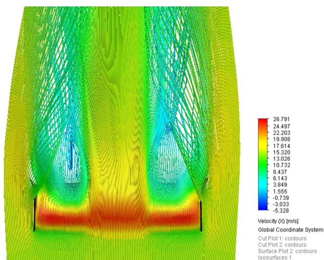
Obr. 44 Vizualizácia prúdenia spodnej strany krídla- pohľad zdola [42]
