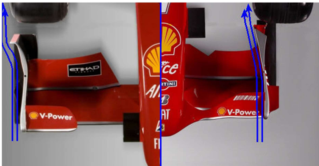
Obr. 37 Znáznornenie prúdenia na endplatoch ( outwash ) na ľavej strane ( inwash ) na pravej [46]
