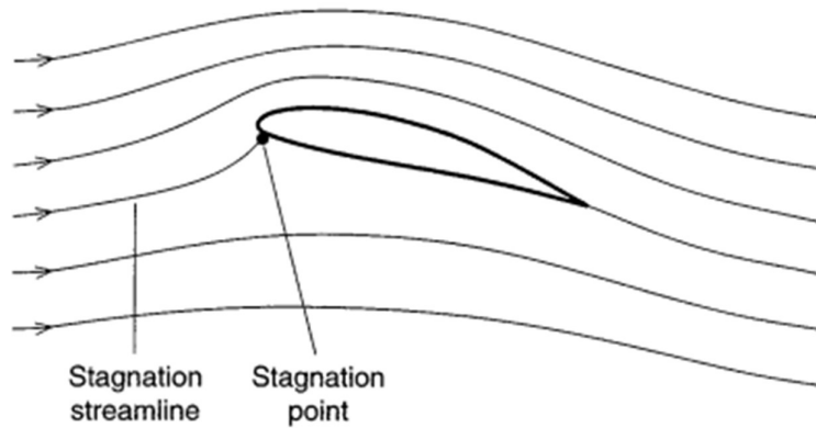
Obr. 9 Prúdové čiary v ustálenom prúde nad krídlom [12]
