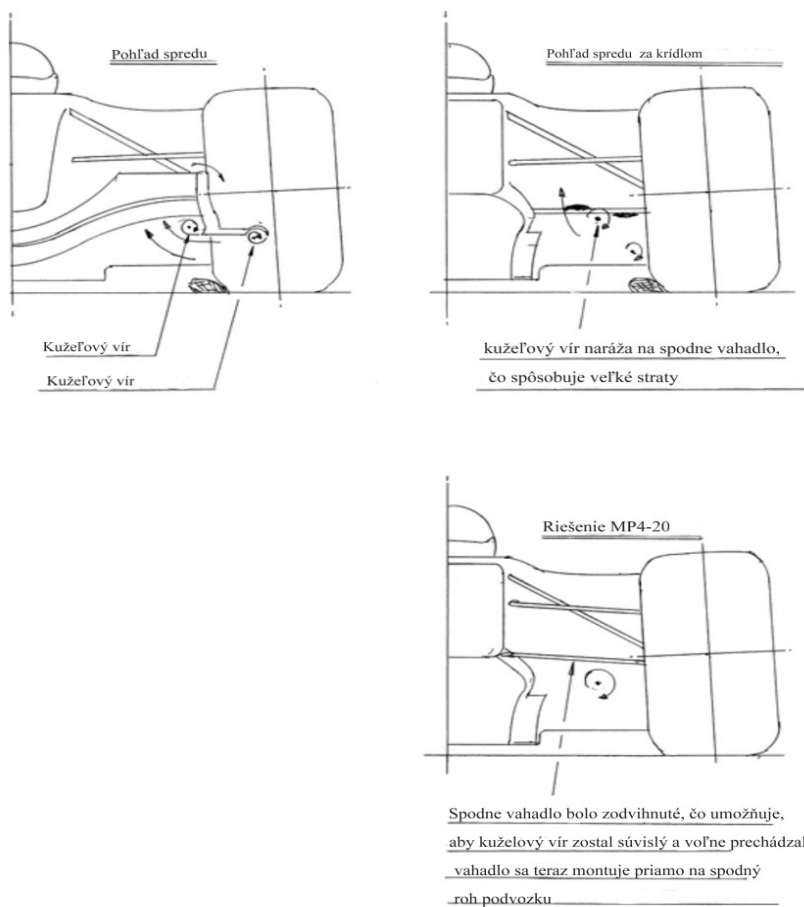
Obr. 23 Riešenie problému s podvozkom [30]
