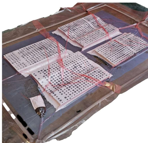
Obr. 70 Ručná laminácia [42]
