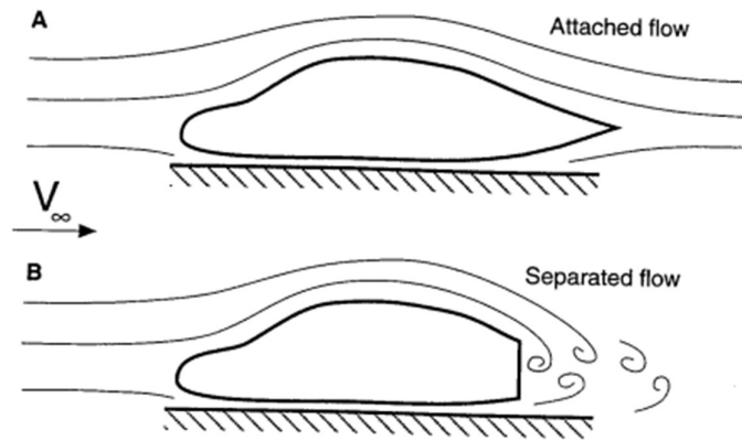
Obr. 7 Vplyv tvaru karosérie na vírenie vzduchu za vozidlom [10]
