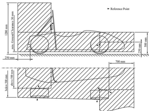
Obr. 34 Stanovené rozmery dané Pravidlami FSG [43]
