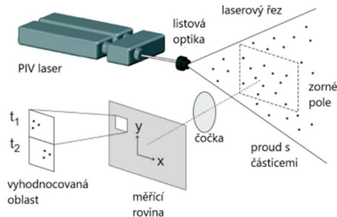
Obr. 81 Schéma a popis zaznamenávania obrazu pomocou PIV [53]
