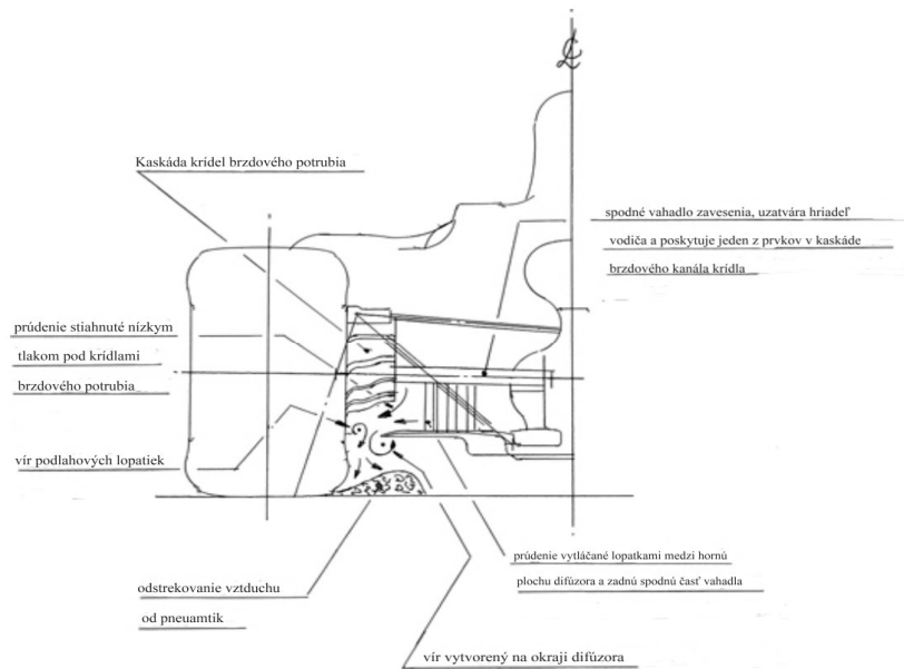
Obr. 25 Optimalizácia zadnej nápravy formule RB8 [32]
