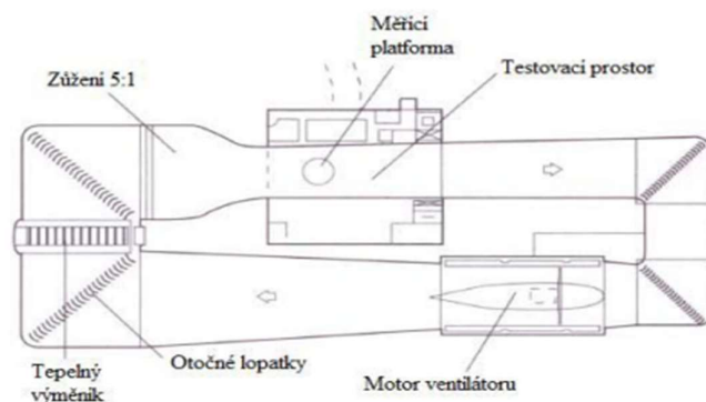
Obr. 29 Aerodynamický tunel s uzavretým okruhom [39]
