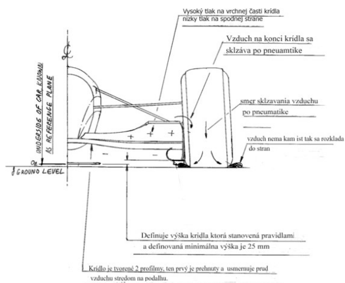
Obr. 20 Technický popis konštrukcie monopostu Williams FW14 [26]
