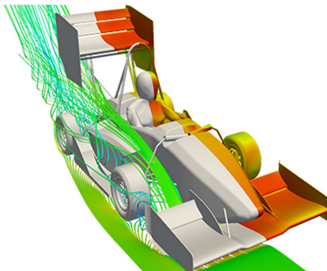
Obr. 30 CFD simulácia [41]
