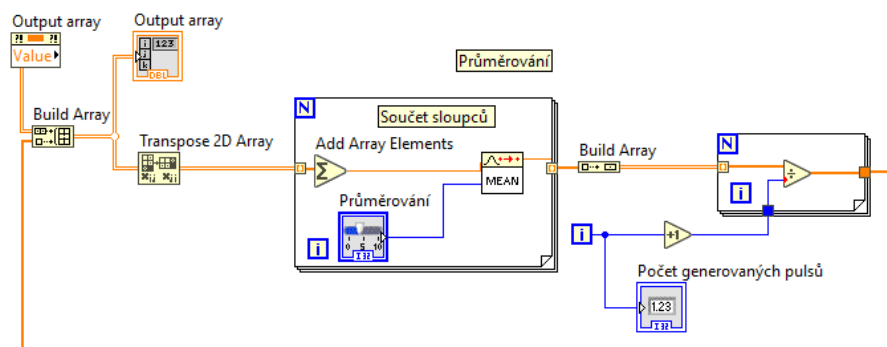
Obr. 7.5: Průměrování pulsu.
