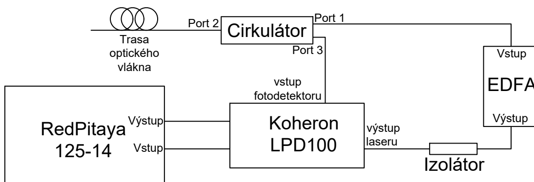
Obr. 6.1: Schéma zapojení.
