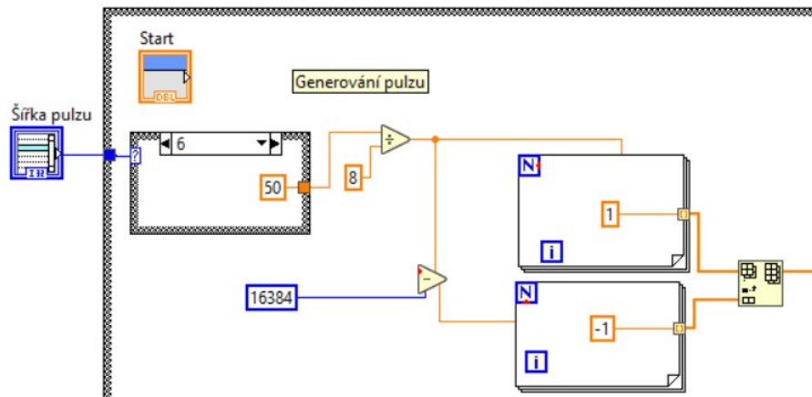
Obr. 7.2: Generování pulsu.
