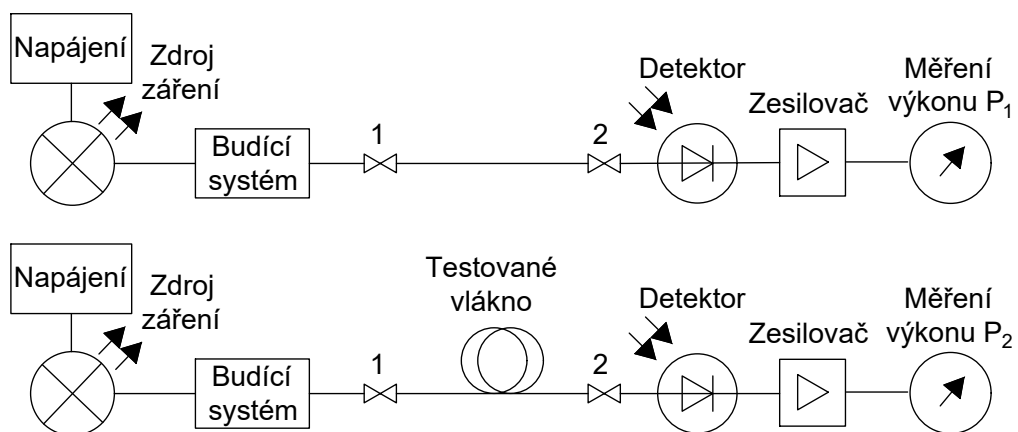
Obr. 1.4: Metoda vložného útlumu [10].
