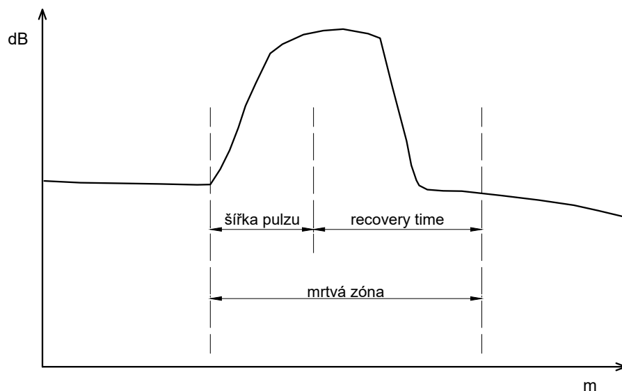
Obr. 4.2: Mrtvá zóna [15].
