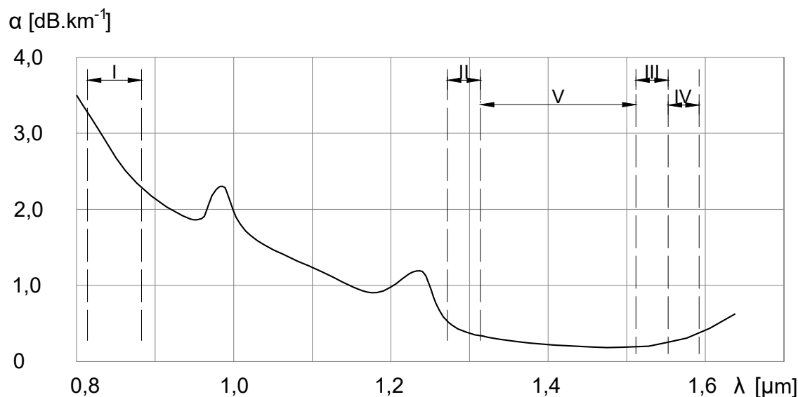
Obr. 5.1: Útlumová charakteristika [15].
