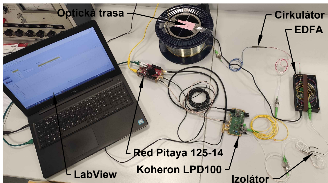
Obr. 9.1: Fotografie zapojení pro metodu měření OTDR.
