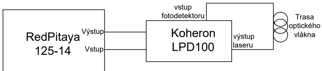
Obr. 10.3: Schéma zapojení pro přímou metodu.
