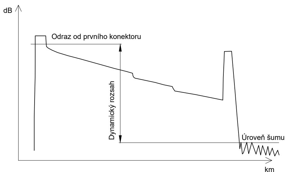
Obr. 4.1: Dynamický rozsah [3].
