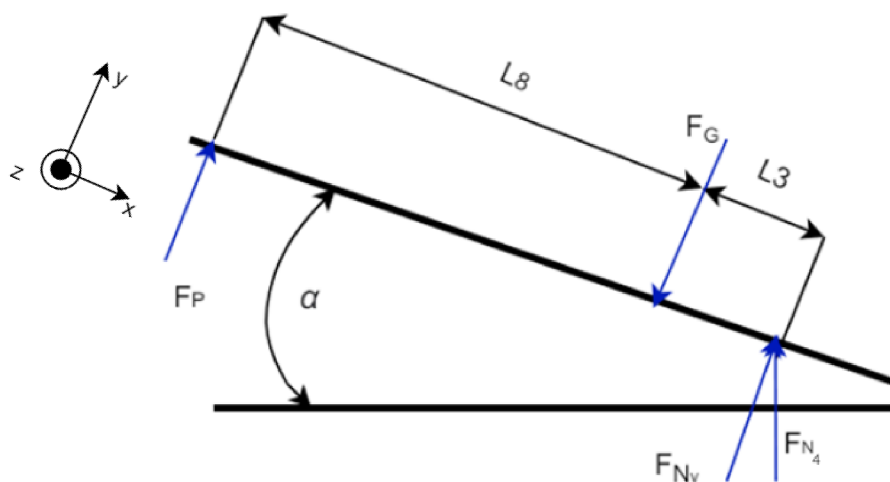
Obr. 53 Zatížení při sklopení návěsu
