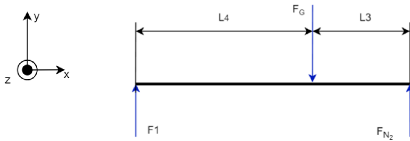
Obr. 43 Zatěžující síly hlavního a tažného rámu
