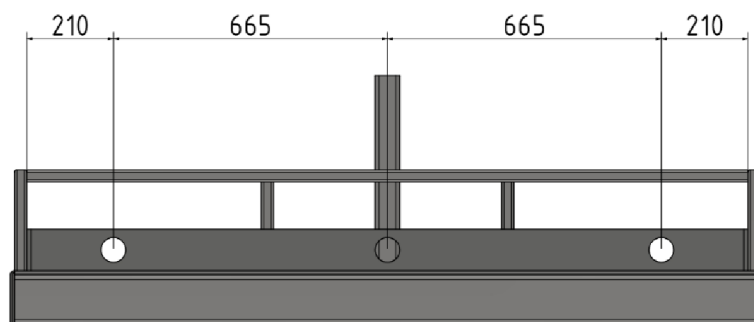
Obr. 32 Rozmístění vazacích bodů v přední části návěsu – z pohledu zezadu
