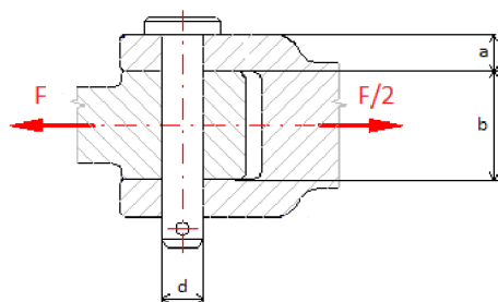
Obr. 48 Obecné schéma zatížení čepu [32]
