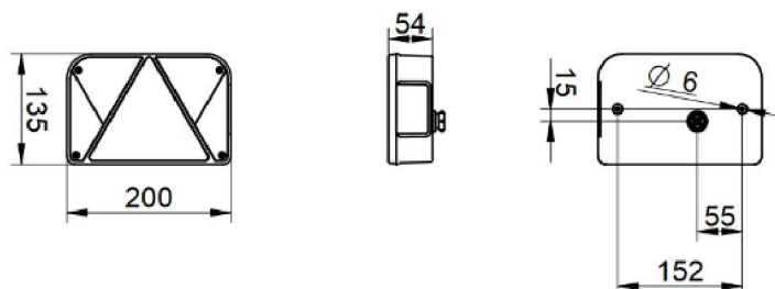
Obr. 33 Koncová svítidla Martz [30]
