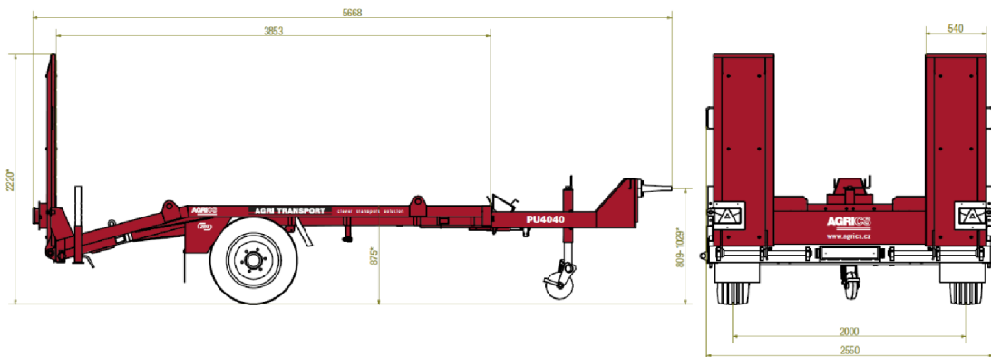
Obr. 5 Podvalník AGRI PU4040 [2]
