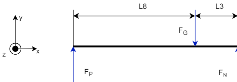
Obr. 54 Zatížení při začátku zvedání návěsu
