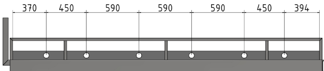
Obr. 31 Rozmístění vazacích bodů na boku návěsu
