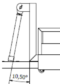
Obr. 55 Zobrazí úhlu uchycení přímočarého hydromotoru
