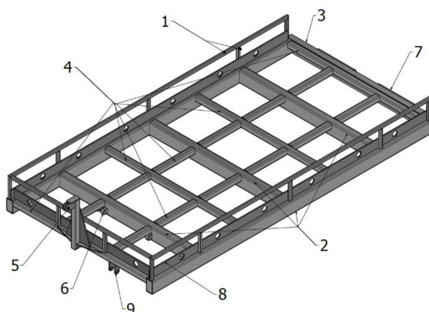
Obr. 24 Hlavní rám - 1- zábradlí, 2 – hlavní nosné příčné a podélné profily, 3 – nosný profil U, 4 - příčné a podélné výztužné profily, 5 – uchycení hydromotoru, 6 – uchycení tažného rámu, 7- uchycení vodící tyče, 8 – ližina uchycení břemene 9 – uchycení čepu pro zajištění rámu
