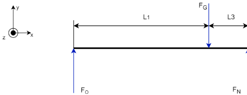
Obr. 39 Působící síly závěsného oka a nápravy
