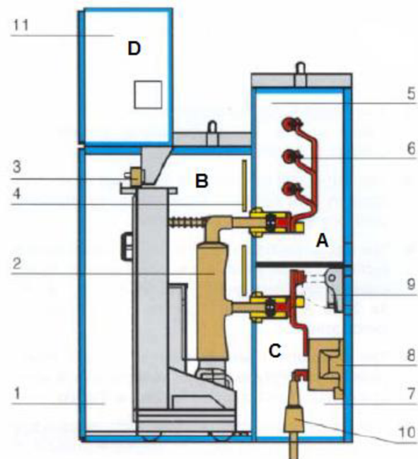
Obr. 5-1: Rez rozvádzačom vn [15]
