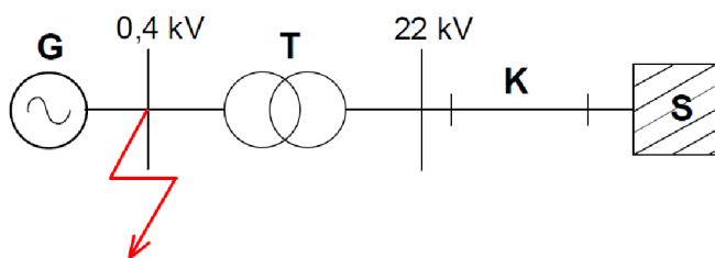
Obr. 6-2: Schéma sústavy pri skrute na rozvádzači nn
