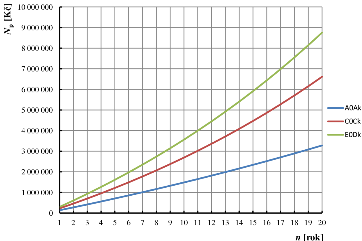
Obr. 3-3: Prevádzkové náklady transformátorov za n rokov
