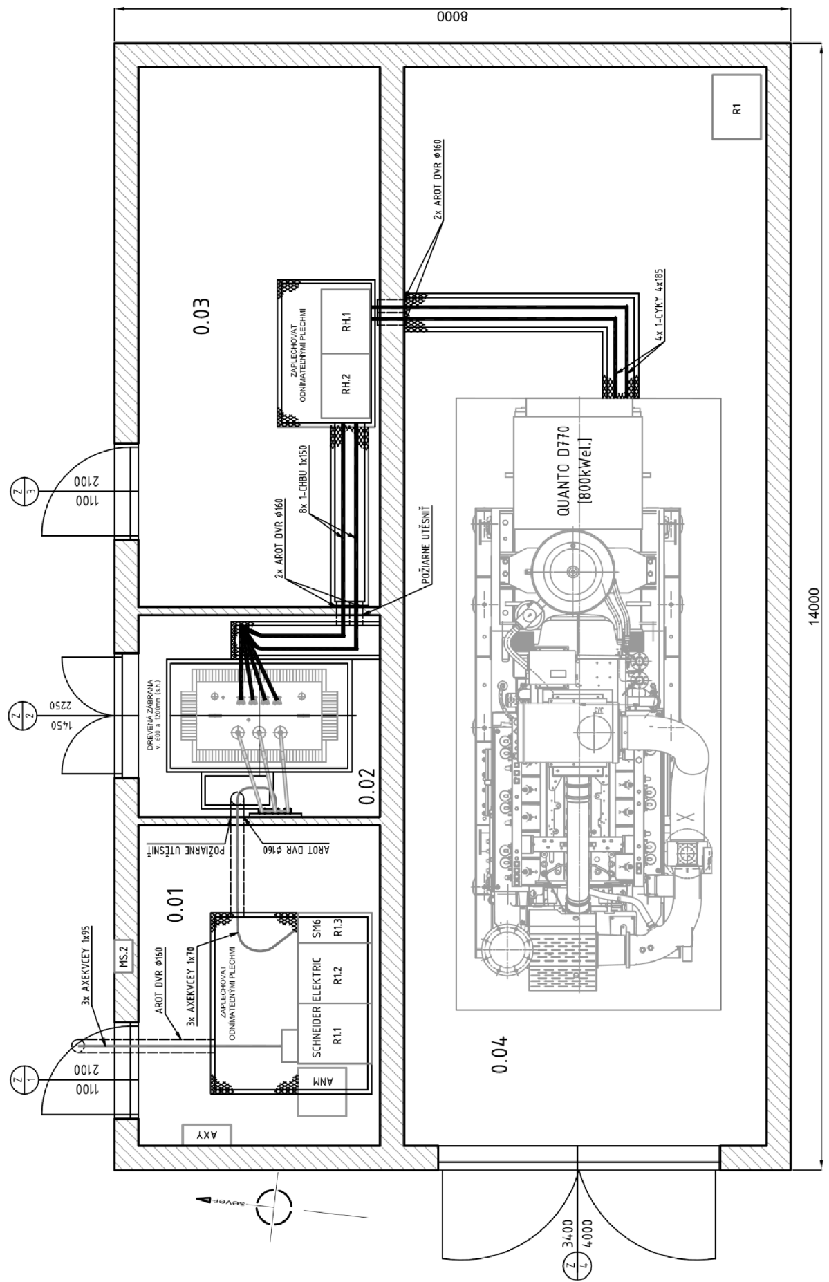
Obr. 7-1: Dispozícia trafostanice
