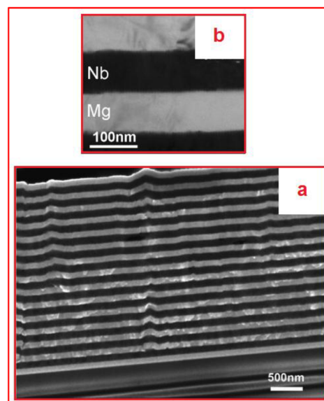
Obr. 2.1.1 Multivrstvý povlak 4. genera- ce, dvojevrstva Mg/Nb, tloušťka 200 nm (a- pohled v řezu, b – zvětšení) 26
