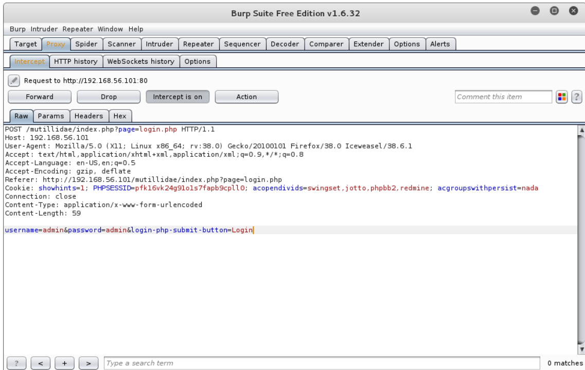
Obr. 4.16: Zachycení HTTP komunikace
