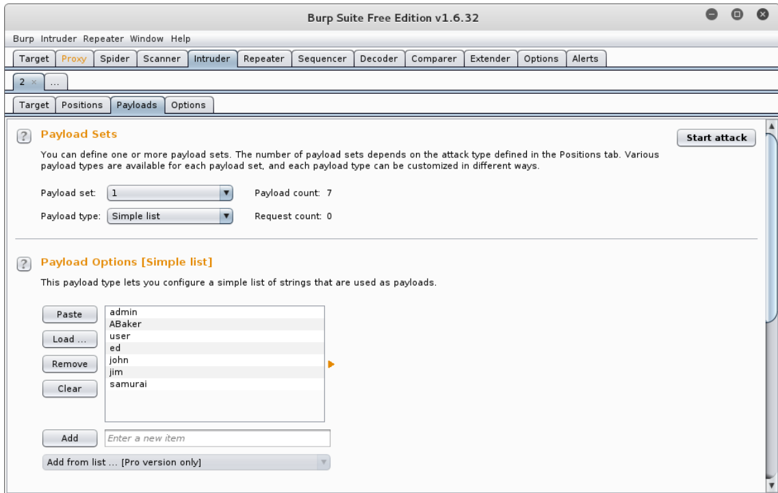
Obr. 4.19: Volba prvních vstupních hodnot (uživatelská jména)
