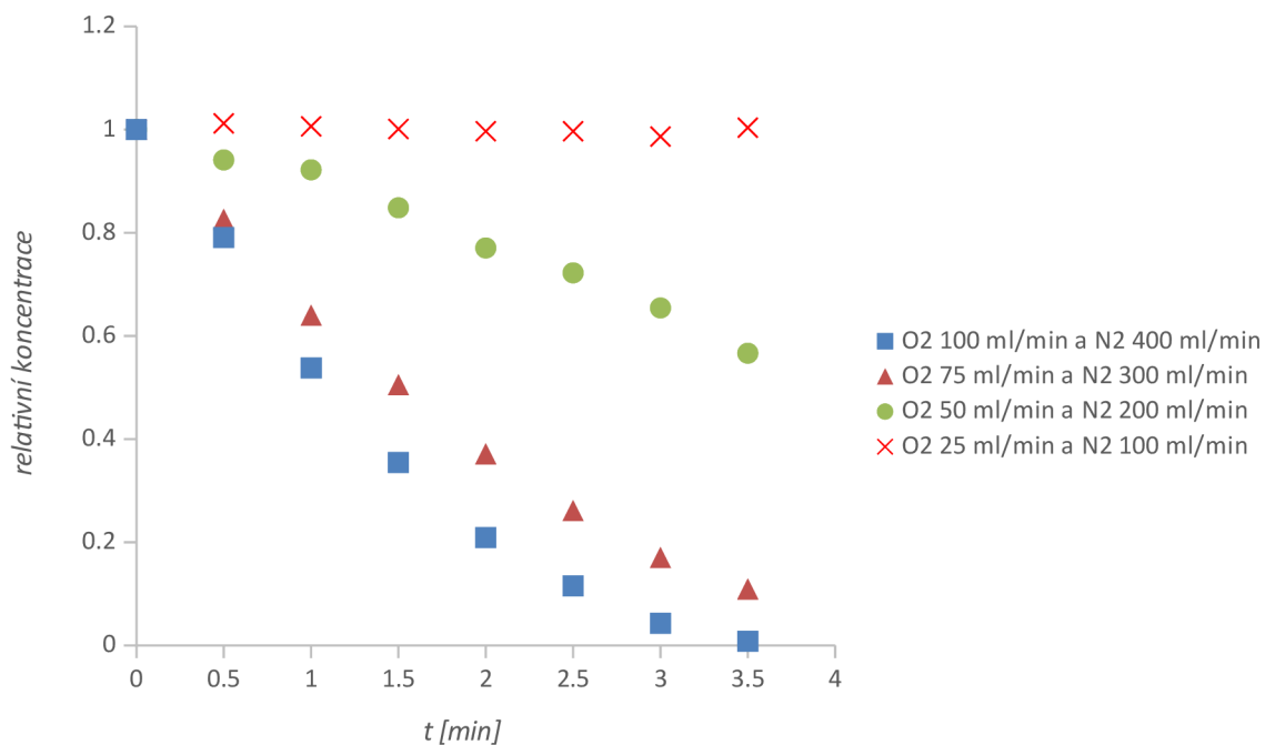
Obrázek 20: Závislost relativní koncentrace roztoku barviva Indigo karmin na čase při zachování poměru průtoku kyslík:dusík 1:4
