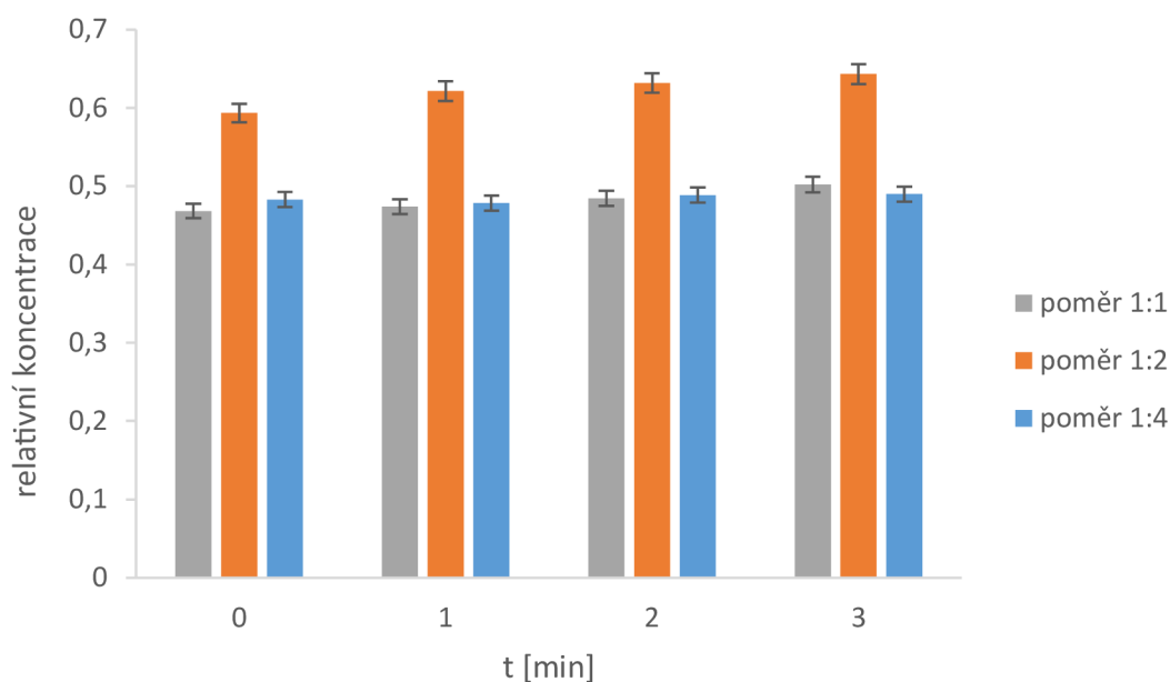
Obrázek 26: Závislost míry odbourání roztoku barviva Saturnová červeň na čase při různém nastavení průtoku plynů kyslík:dusík
