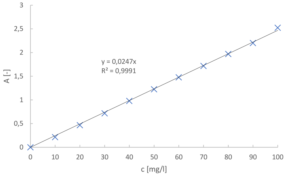
Obrázek 15: Závislost absorbance vzorku barviva Saturnová červeň na koncentraci
