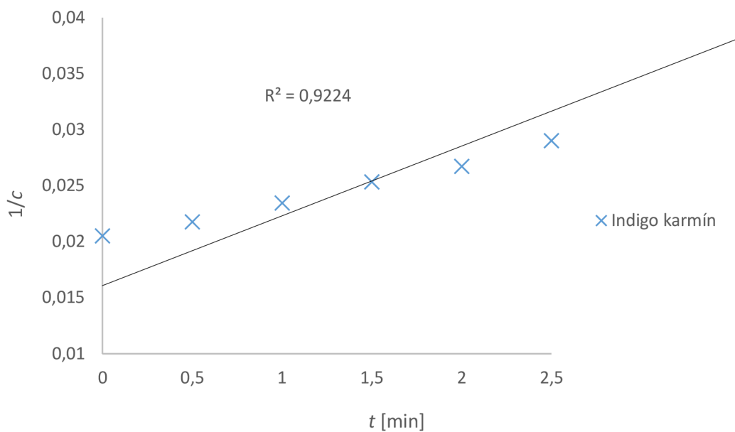
Obrázek 33: Závislost převrácené koncentrace barviva Indigo karmín na čase pro průtok O_2 50 ml/min a N_2 100 ml/min
