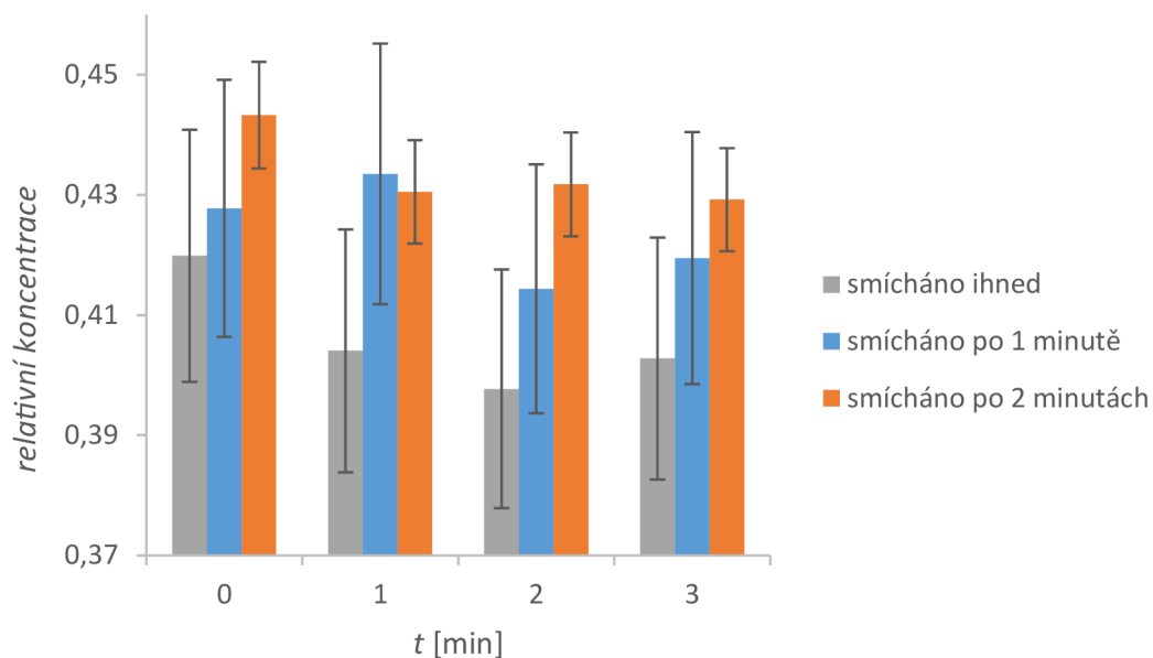
Obrázek 25: Závislost relativní koncentrace barviva Indigo karmín na čase a době uplynulé mezi výrobou PAW a smíchání se vzorkem barviva pro nastavení průtoků plynů v poměru 1:1, doba výroby 5 minut
