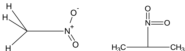
Obrázek č.7: Strukturální vzorce nitrometanu a nitropropanu (vytvořeno autorem)
