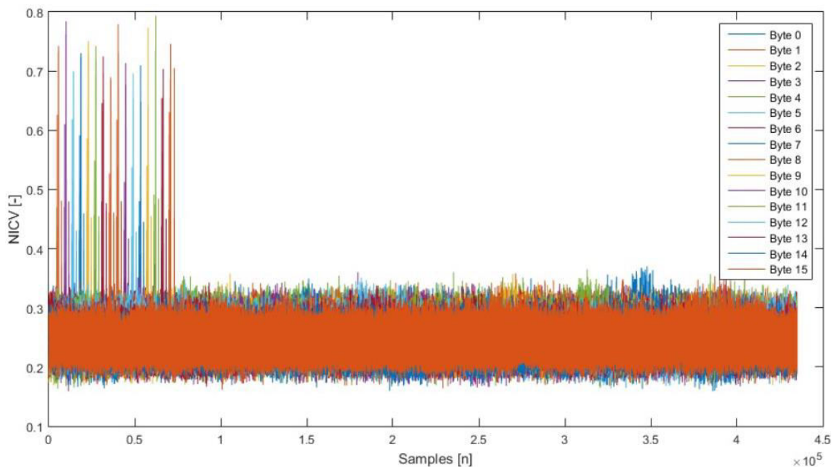
Obr. 4.2.3: NICV počítáno pro 1000 průběhů proudové spotřeby
