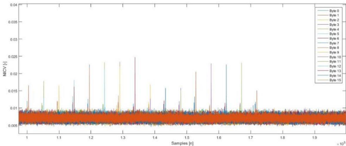
Obr. 4.2.2: Přibližné malé špičky odpovídající operaci SubBytes
