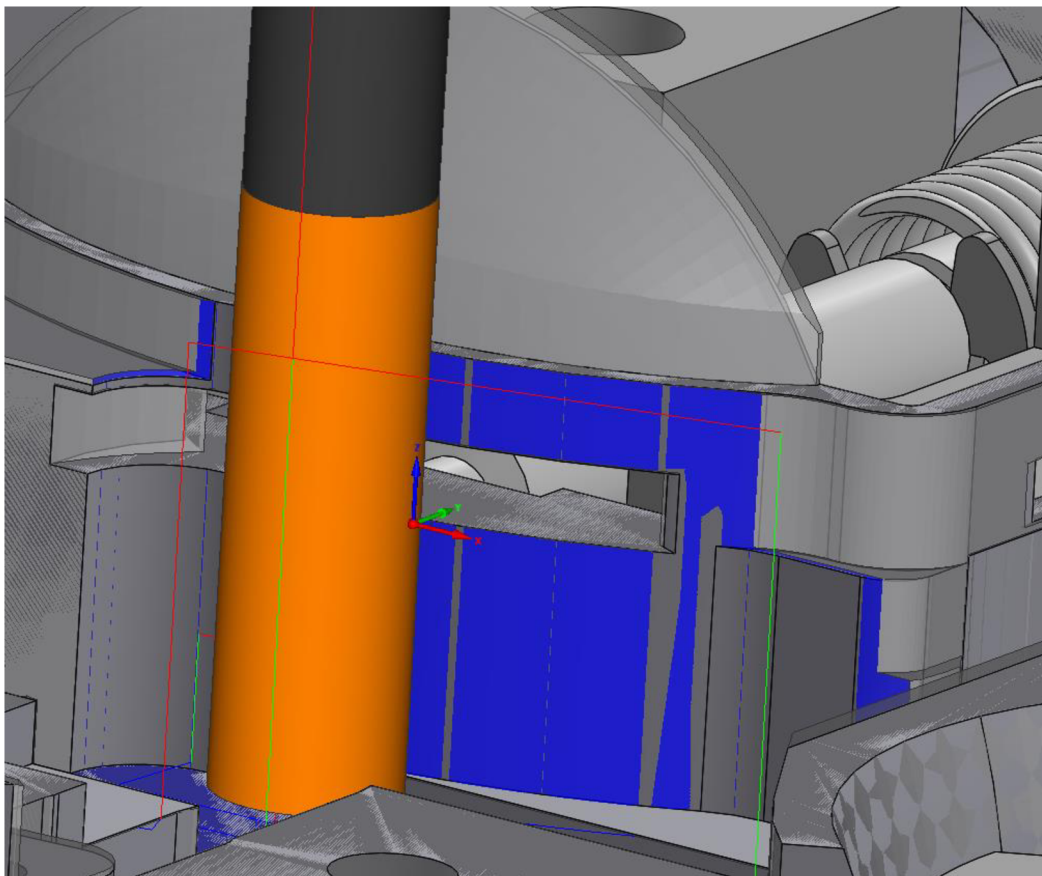
Obr. 38 Frézování bokem válcové čelní frézou.
