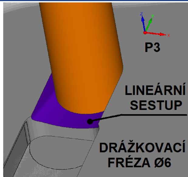
Obr. 12 Postupné zahlubování po lineární dráze.
