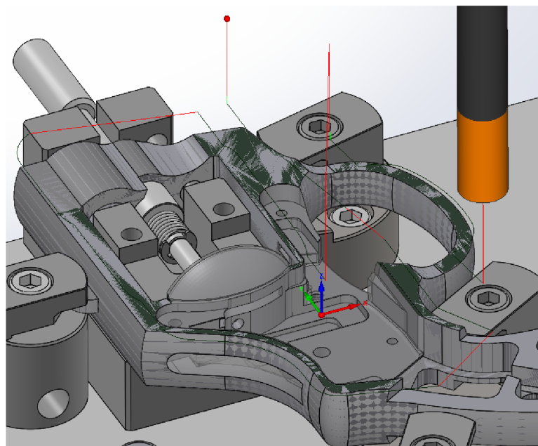
Obr. 37 Dokončování výměnitelnou hlavicí Ø12.
