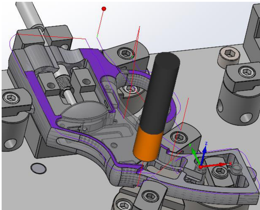
Obr. 36 Hrubování čelní frézou s VBD Ø16 pro vysoké posuvy.
