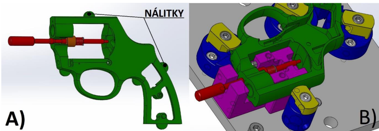
Obr. 8 A) Ustavení trnu, B) osazení do upínače.
