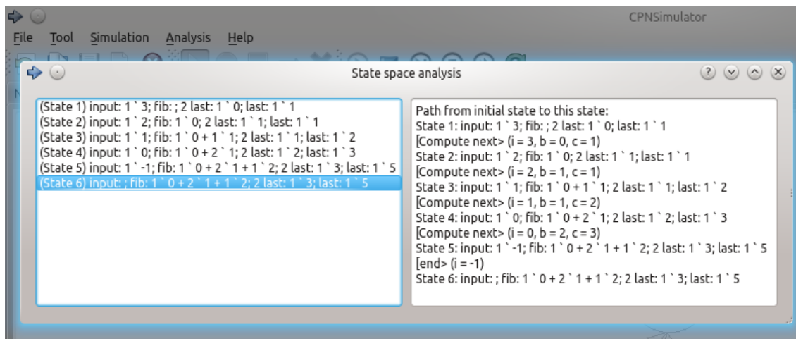
Obrázek 6.10: Modální okno průzkumníka grafu dosažitelných značení
