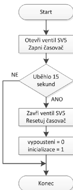
Obr. 47: Vývojový diagram funkce Vypoustení
