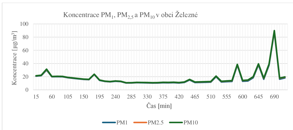
Obrázek 29: Koncentrace PM 1 , PM 2,5 a PM 10 v obci Železné.
