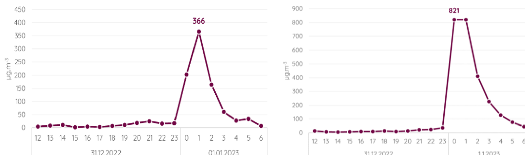
Obrázek 57: Vlevo graf koncentrace částic PM 10 při ohňostrojích pro Prahu a vpravo pro Tábor [22].
