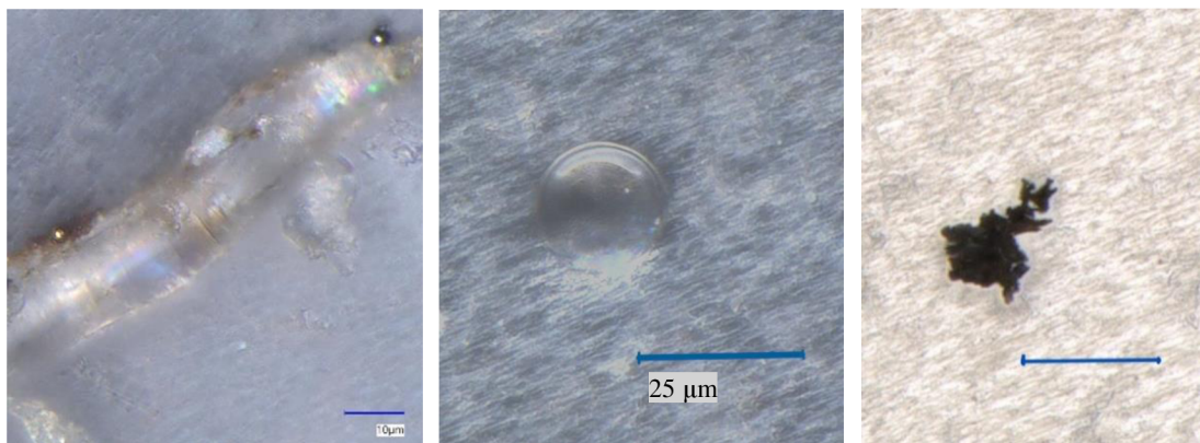
Obrázek 27: Venkovské imise.
