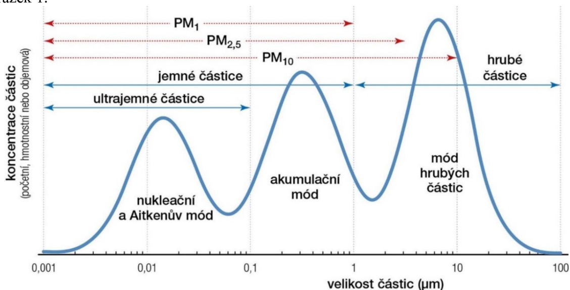
Obrázek 1: Koncentrace částic v závislosti na velikosti, velikostní kategorie [2].
