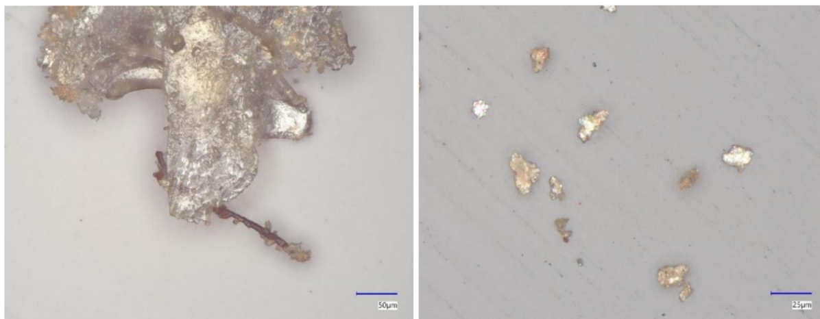
Obrázek 37: Imisní odběr v domě, obří částice s krystaly a kusem vlákna a oblast s částicemi o velikosti jednotek až desítek mikrometrů.
