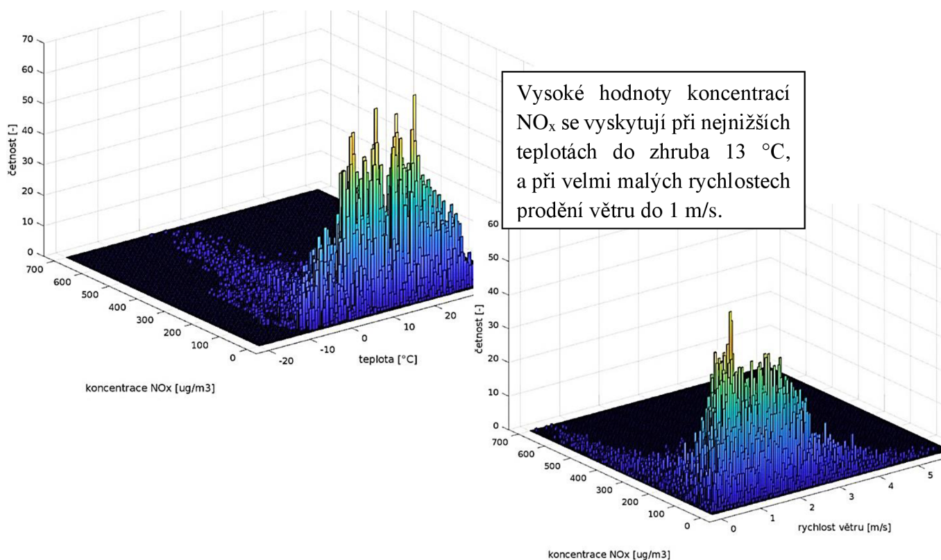
Obrázek 44: Grafy koncentrací NO x v závislosti na teplotě a rychlosti větru a četnosti měření.
