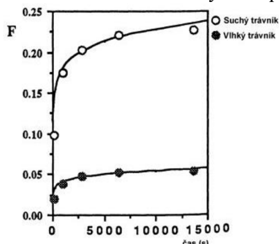
Obrázek 4: Podíl částic zviřených prouděním vzduchu nad travnatým povrchem [13].
