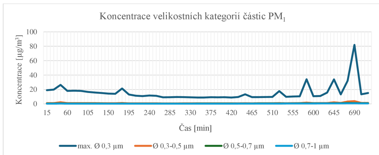
Obrázek 30: Koncentrace velikostních kategorií částic PM_{10} v obci Železná.
