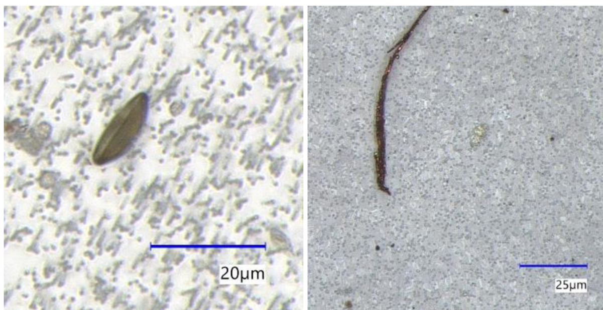
Obrázek 31: Městské imise.
