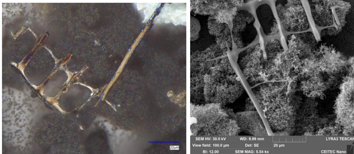
Obrázek 16: Úlet z komínu z dilenských kamen, netypická částice, vlevo pod optickým mikroskopem, vpravo pod elektronovým mikroskopem.
