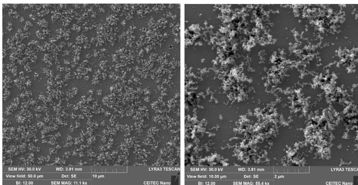
Obrázek 19: Výfukové emise, měřítko 10 a 2 µm, elektronový mikroskop.
