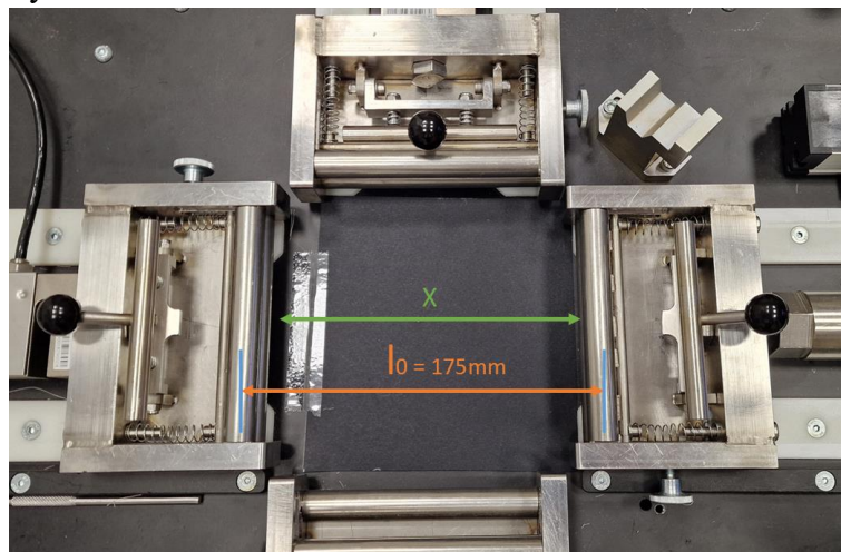
Obrázek 25 Směr zatěžování a upínací délka
