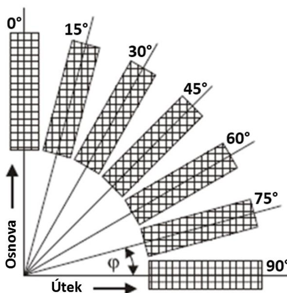
Obrázek 20 Úhly odebíraných vzorků
