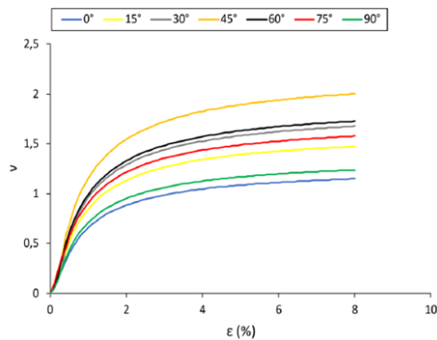
Obrázek 14 Poissonův poměr tkanin v atlasové vazbě (24)
