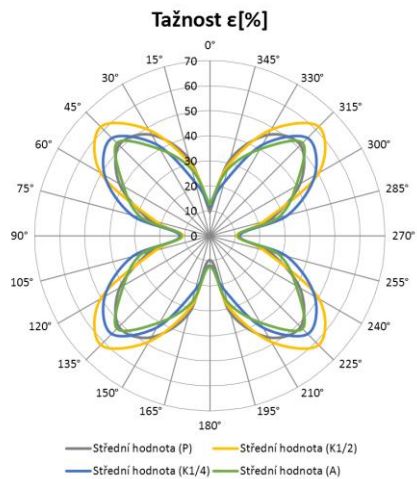
Obrázek 66 Výsledný diagram Tažnosti (bez intervalů)
