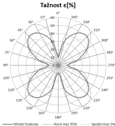
Obrázek 48 Tažnost plátňové vazby
