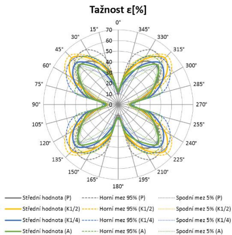
Obrázek 65 Výsledný diagram Tažnosti
