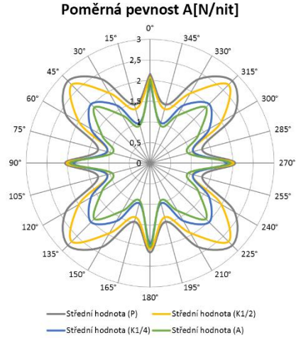
Obrázek 64 Výsledný diagram Poměrné pevnosti (bez intervalů)
