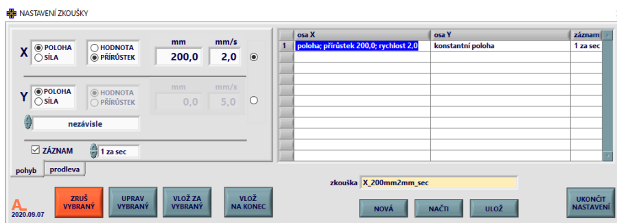
Obrázek 36 Nastavení parametrů tahové zkoušky
