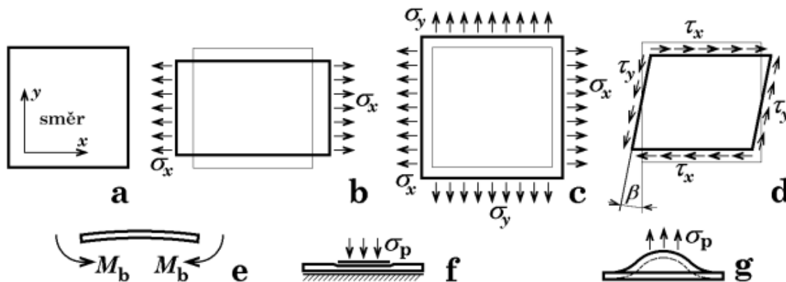
Obrázek 5 Formy rovinné deformace a,b) Jednoosé zatížení, c) Biaxiální napětí, d) Smykové napětí, e) Ohybové napětí, f) Příčné stlačení, g) vyboulení textilie (7)
