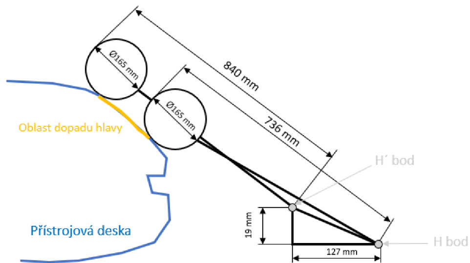
Obr. 57 Určení dopadu hlavy – zdroj autor
