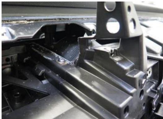
Obr. IV Přístrojová deska po zkoušce číslo 2 – zdroj autor
