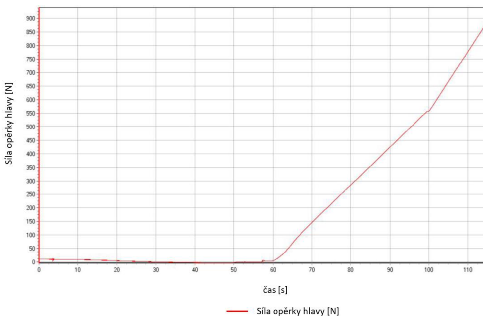
Graf 4 Síla působící na hlavovou opěrku silou max. 890 Nm – zdroj autor
