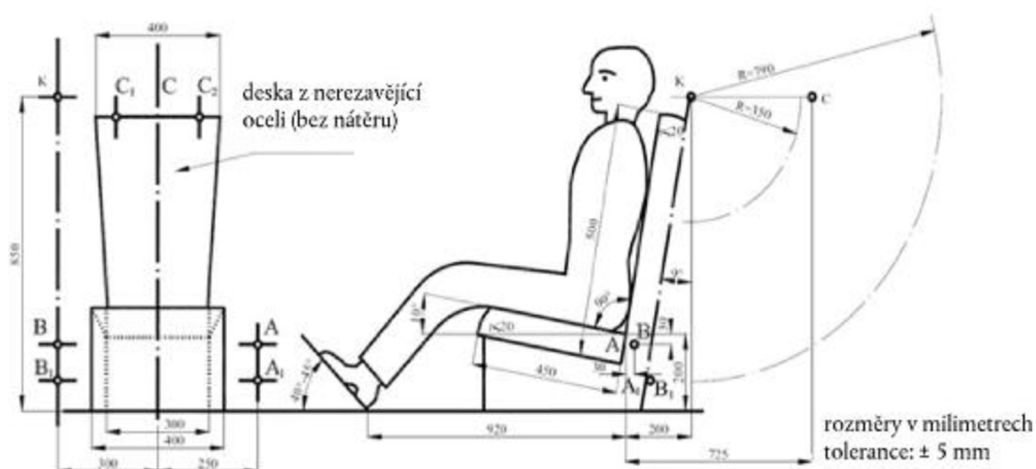
Obr. 12 Zkouška na zkušebním vozíku dle OSN č.16 (9)
