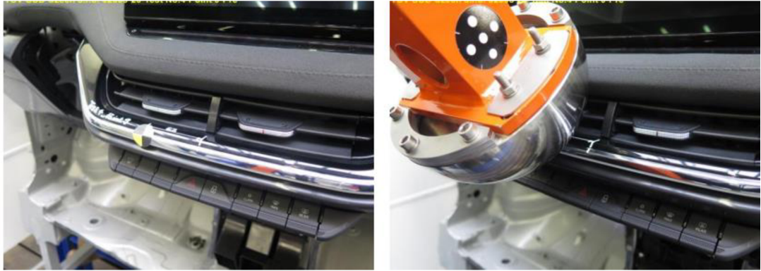
Obr. IV Přístrojová deska před zkouškou číslo 4– zdroj autor
