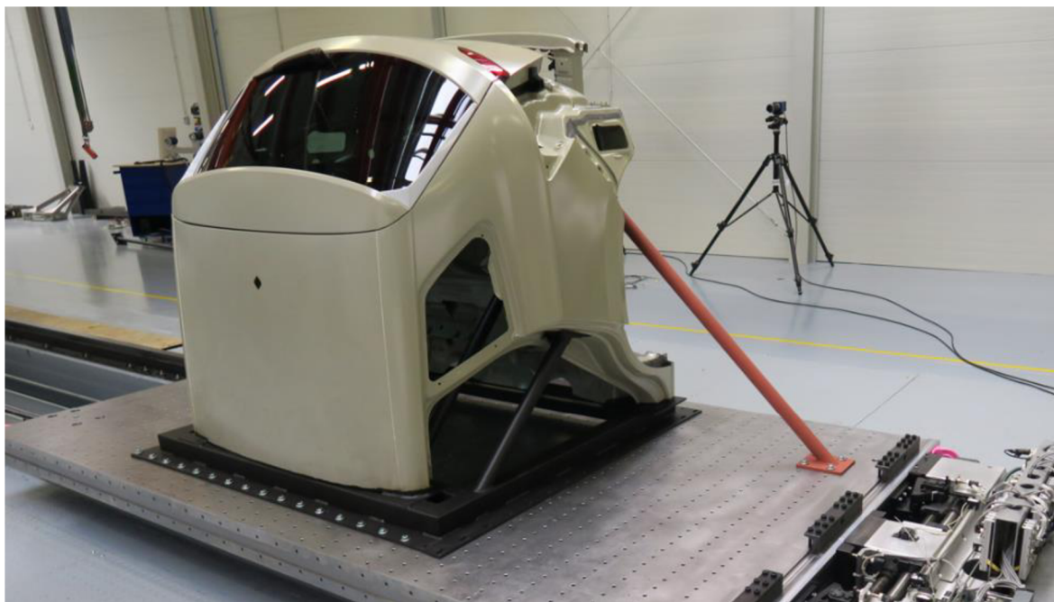
Obr. 6 Zkouška pevnosti upevnění dveří – zdroj autor
