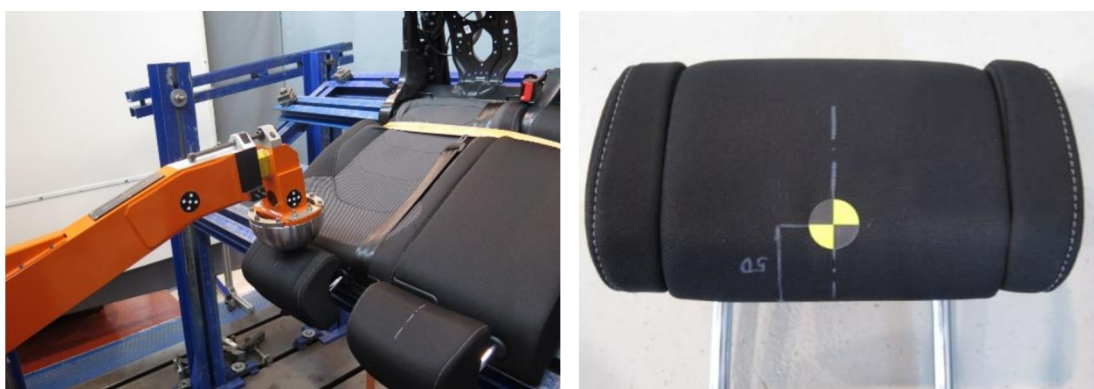
Obr. 80 Zkouška pohlcení energie hlavové opěrky zepředu druhá řada – zdroj autor
