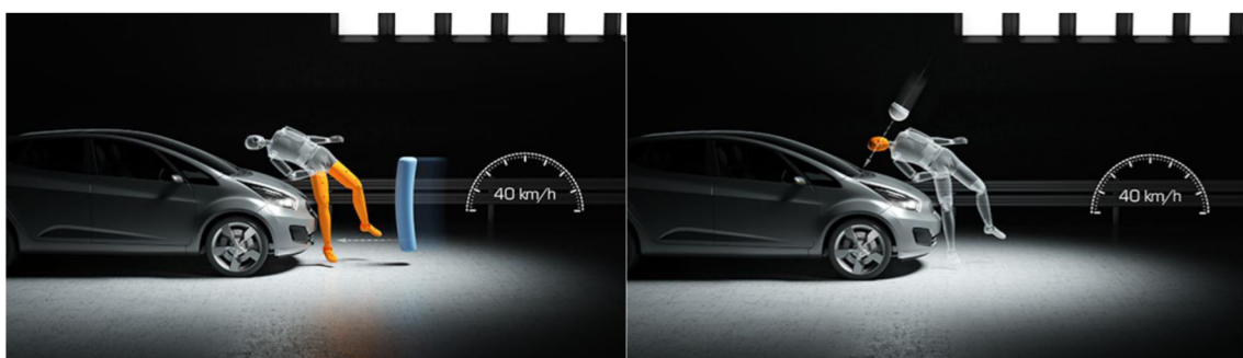
Obr. 28 Znárodnění testů pro ochranu chodců (25)
