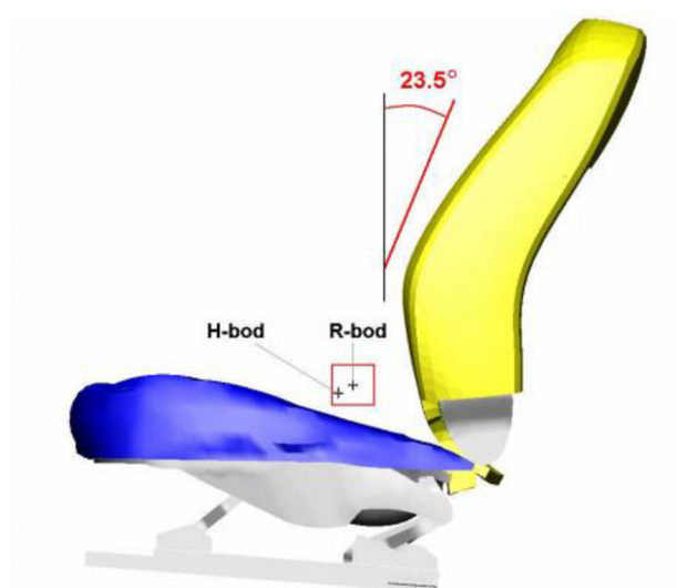
Obr. 66 Ukázka polohy H-bodu vůči R-Bodu (40)
