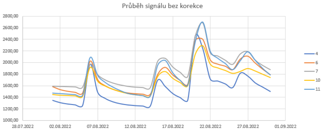
Obrázek 5.11 – Průběh signálu bez korekce
