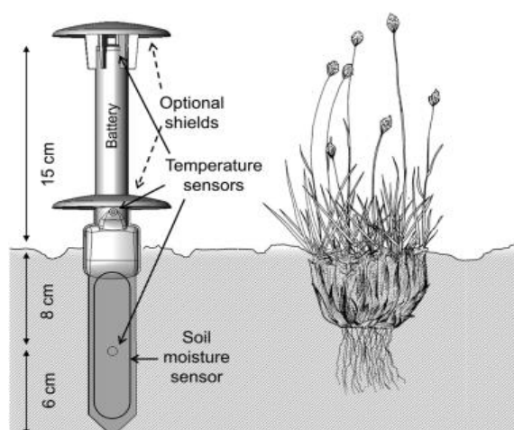
Obrázek 5.5 – Schéma TMS senzoru s popisem rozmístění teploměrů a vlhkostního senzoru (Wild et al., 2019)
