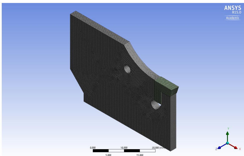
Obr. 2.14 Zasíťovaný model.
