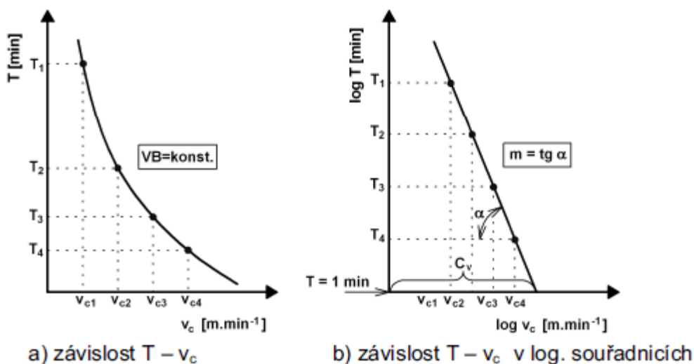
Obr. 1.17 T-v_c závislost [7].
