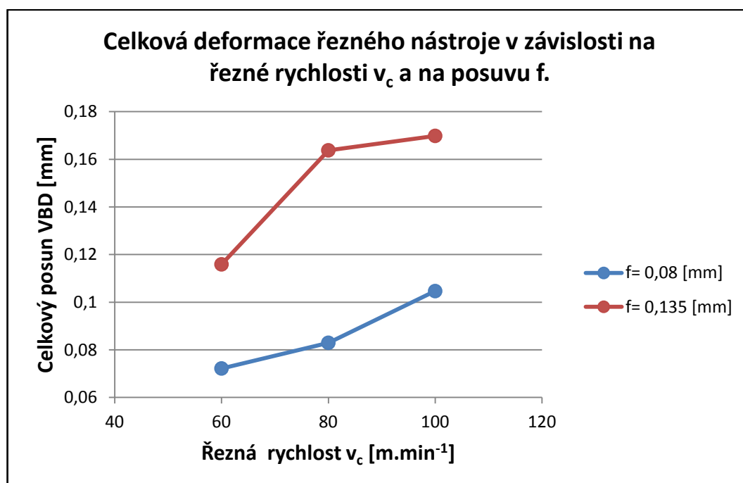
Obr. 2.24 Celková deformace.
