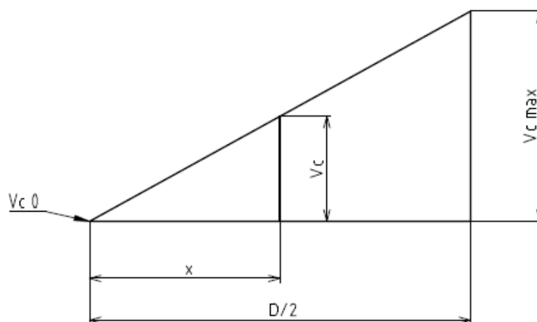
Obr. 1.6 Rovnost trojúhelníků.
