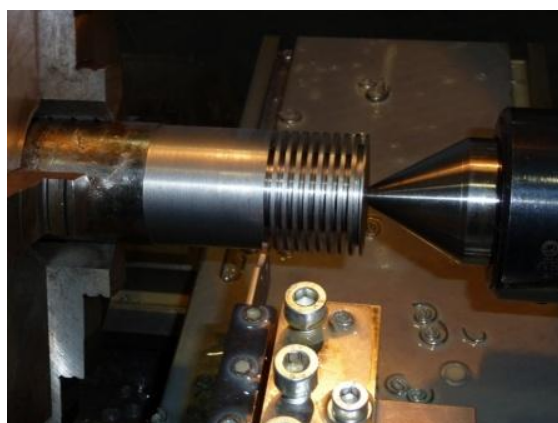
Obr. 2.6 Jednotlivé experimentální zápichy do zkušebního vzorku.
