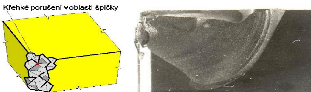
Obr. 1.14 Schéma a fotografie křehkého porušení v oblasti špičky [7].
