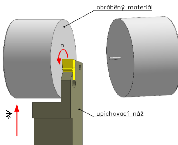
Obr. 1.1 Schéma upichování [3].
