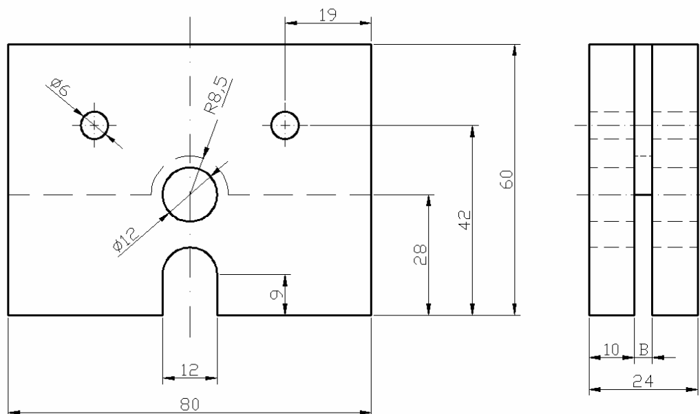
Obr. 6.10: Experimentální přípravek zkonstruovaný pro přesné vedení vzorků při zkoušce lomové houževnatosti
