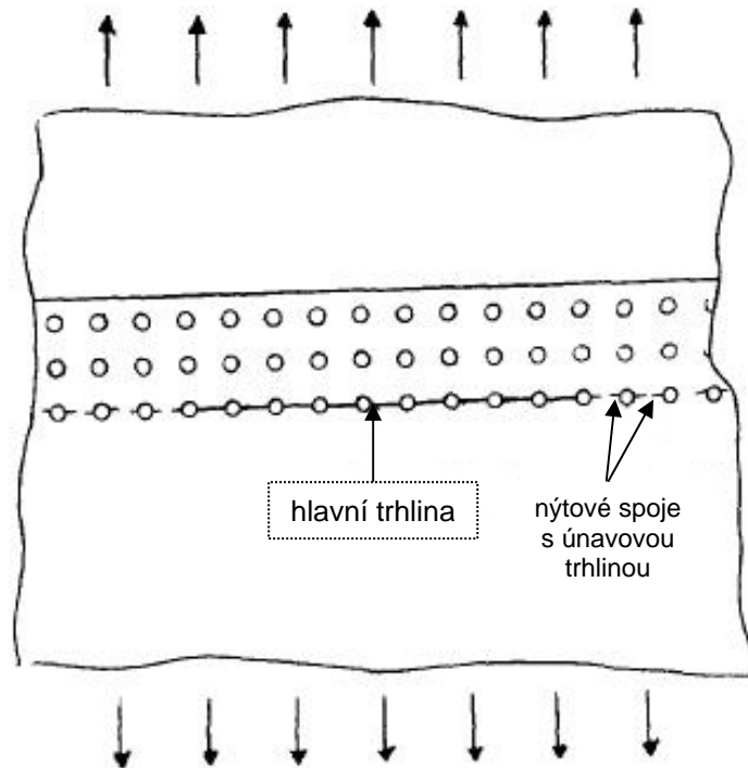
Obr. 4.11: Nýtované spoje duralových plechů v geometrickém uspořádání, které způsobuje nízkou lomovou odolnost součásti [22]
