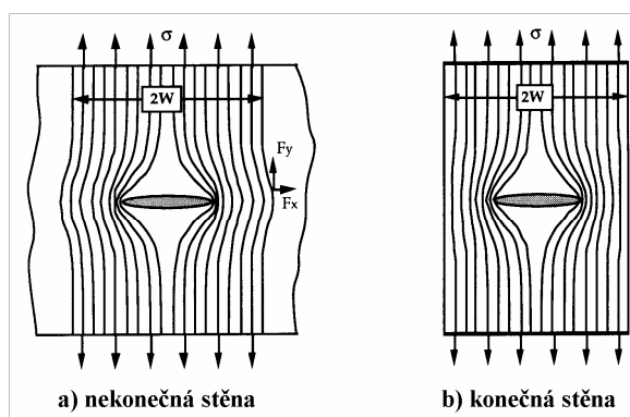
Obr. 3.2: Koncentrovaná napětí v okolí ostré trhliny [1]
