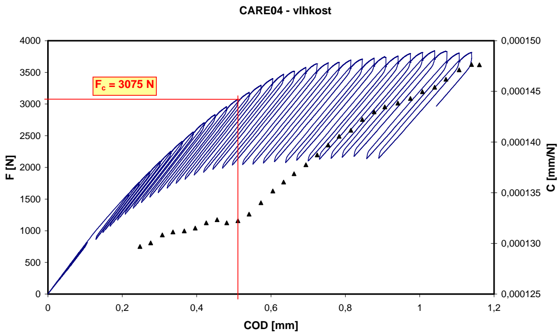
Obr. 6.20: Závislost změny síly a poddajnosti na změně rozevření trhliny VKL CARE04 ovlivněného absorbovanou vlhkostí
