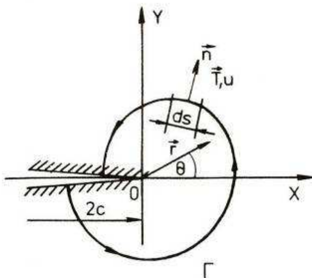
Obr. 3.20: Grafické znázornění J integrálu, c = a [24]
