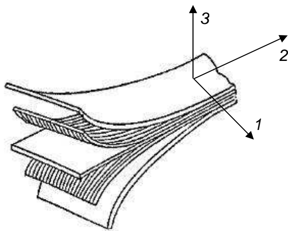
Obr. 4.9: Jednosměrné uspořádání VKL [5]
