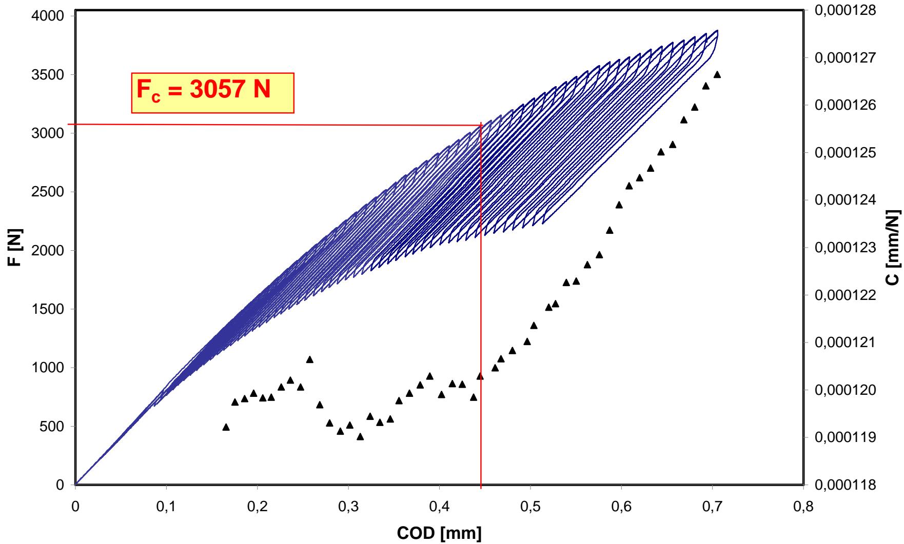
Obr. 6.15: Závislost změny síly a poddajnosti na změně rozevření trhliny VKL CARE07
