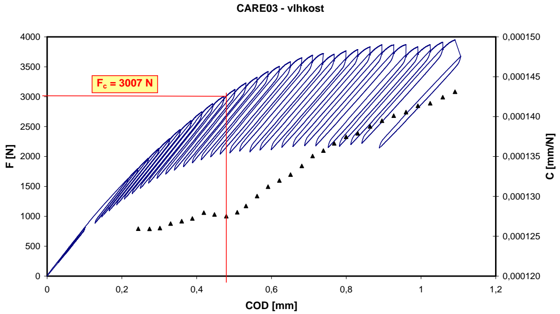
Obr. 6.19: Závislost změny síly a poddajnosti na změně rozevření trhliny VKL CARE03 ovlivněného absorbovanou vlhkostí
