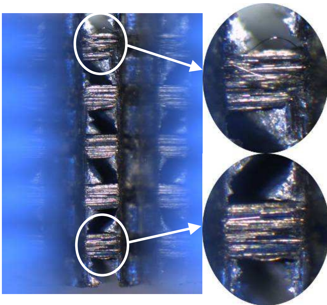
Obr. 6.33: Detailní zobrazení rozevřené trhliny vzniklé po “kolapsu“ VKL způsobeném přetržením většího počtu uhlíkových vláken v krajních vrstvách; CARE05
