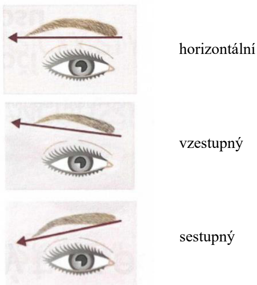
Obr. 7: Typy obočí
