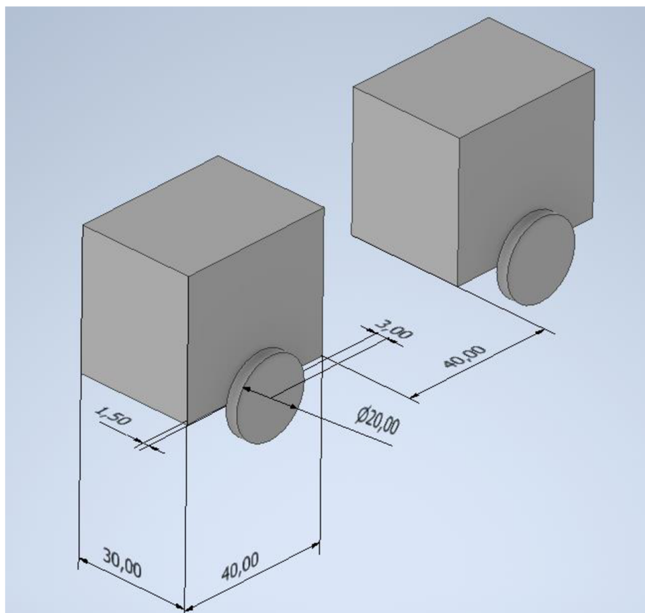
Obr. 24 Rozmery jedného článku
