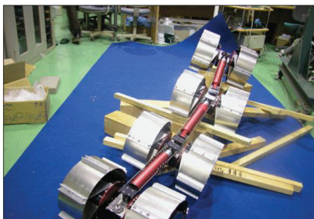
Obr. 14 Genbu [8]
