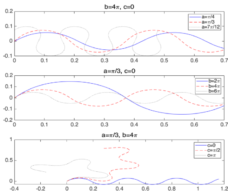
Obr. 6 Grafický priebeh vplyvov konštánt a, b, c [9]
