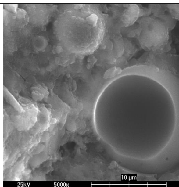
Geopolymer CH25A1,0 zvětšeno 5000x
