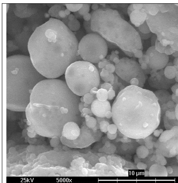
Popílek Chvaletice - zvětšeno 5000x
