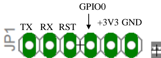
Obr. 21 Rozložení pinů na programovacím konektoru lokalizačního zařízení
