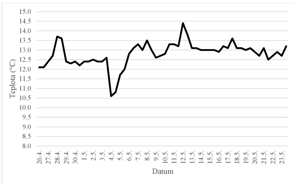
Graf 1 Teplota vody v průběhu experimentu
