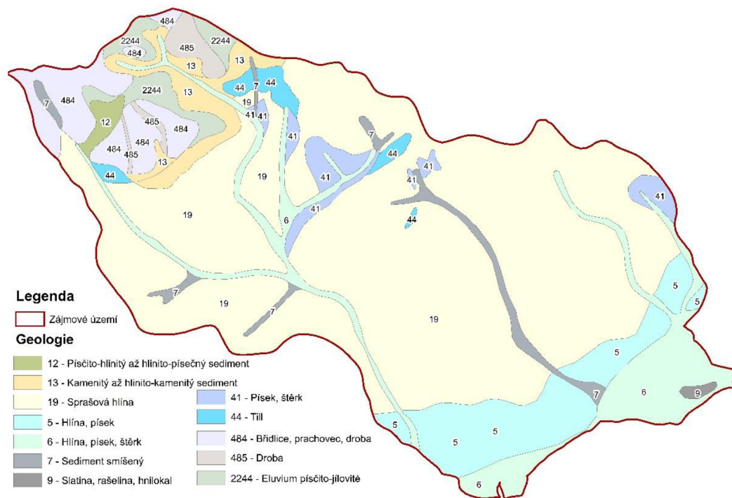
Obrázek 3.1 - Geologické podmínky
