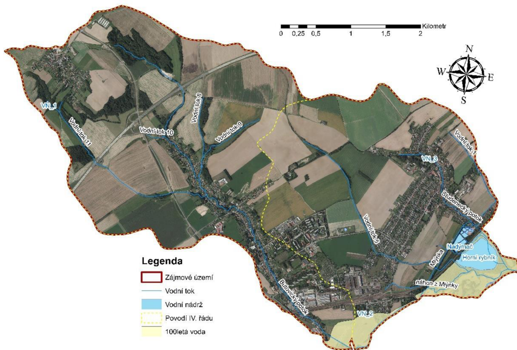
Obrázek 3.3 - Hydrologické podmínky
