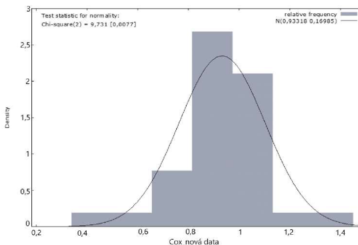
Obrázek 21 – Histogram rozložení dat – obsah org. uhlíku (v %) nová data
