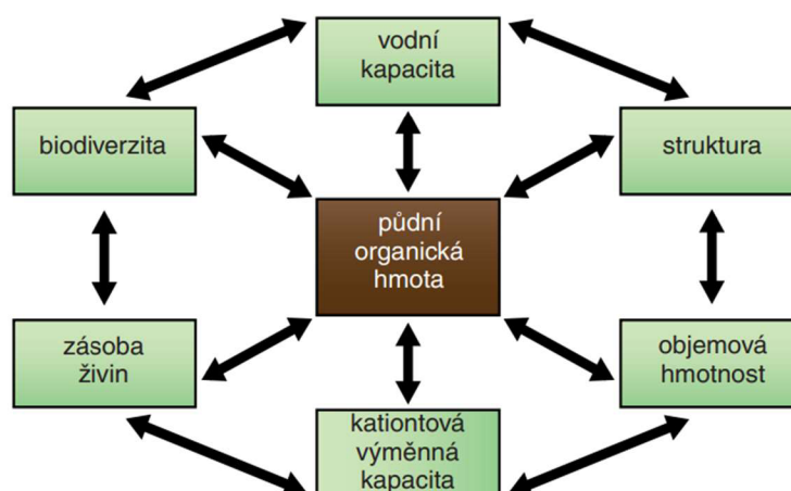
Obrázek 1 – Vztah mezi půdní organickou hmotou a dalšími důležitými charakteristikami a funkcemi půdy, zdroj: Šimek a kol., 2021
